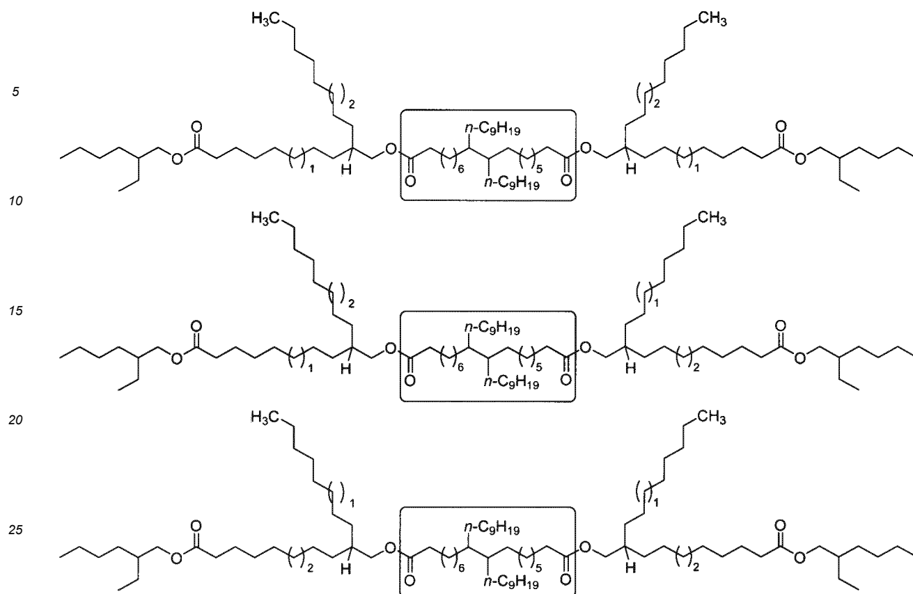
Abbildung 9. Besonders bevorzugter Vertreter der erfindungsgemäßen Verbindungen gemäß der bevorzugten allgemeinen Struktur (Ic), hergestellt ausgehend von der Dicarbonsäure Pripol 1013 als Dicarbonsäure-Komponente
