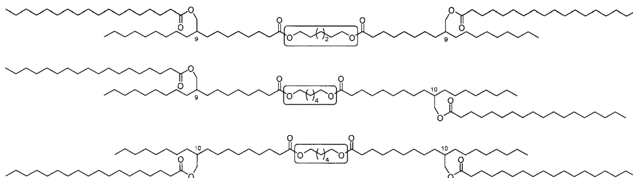
Abbildung 7. Besonders bevorzugter Vertreter der erfindungsgemäßen Verbindungen gemäß der bevorzugten allgemeinen Struktur ( 1b ), hergestellt ausgehend von 1,6-Hexandiol als Diol-Komponente
