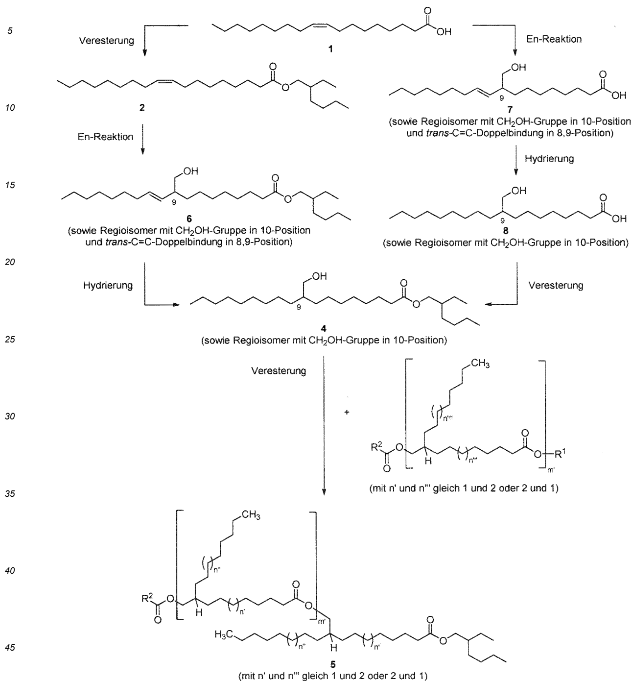
Abbildung 6. Bevorzugte Synthesestrategien ausgehend von Ölsäure und unter Einbezug einer En-Reaktion zur Herstellung von Verbindungen 5
