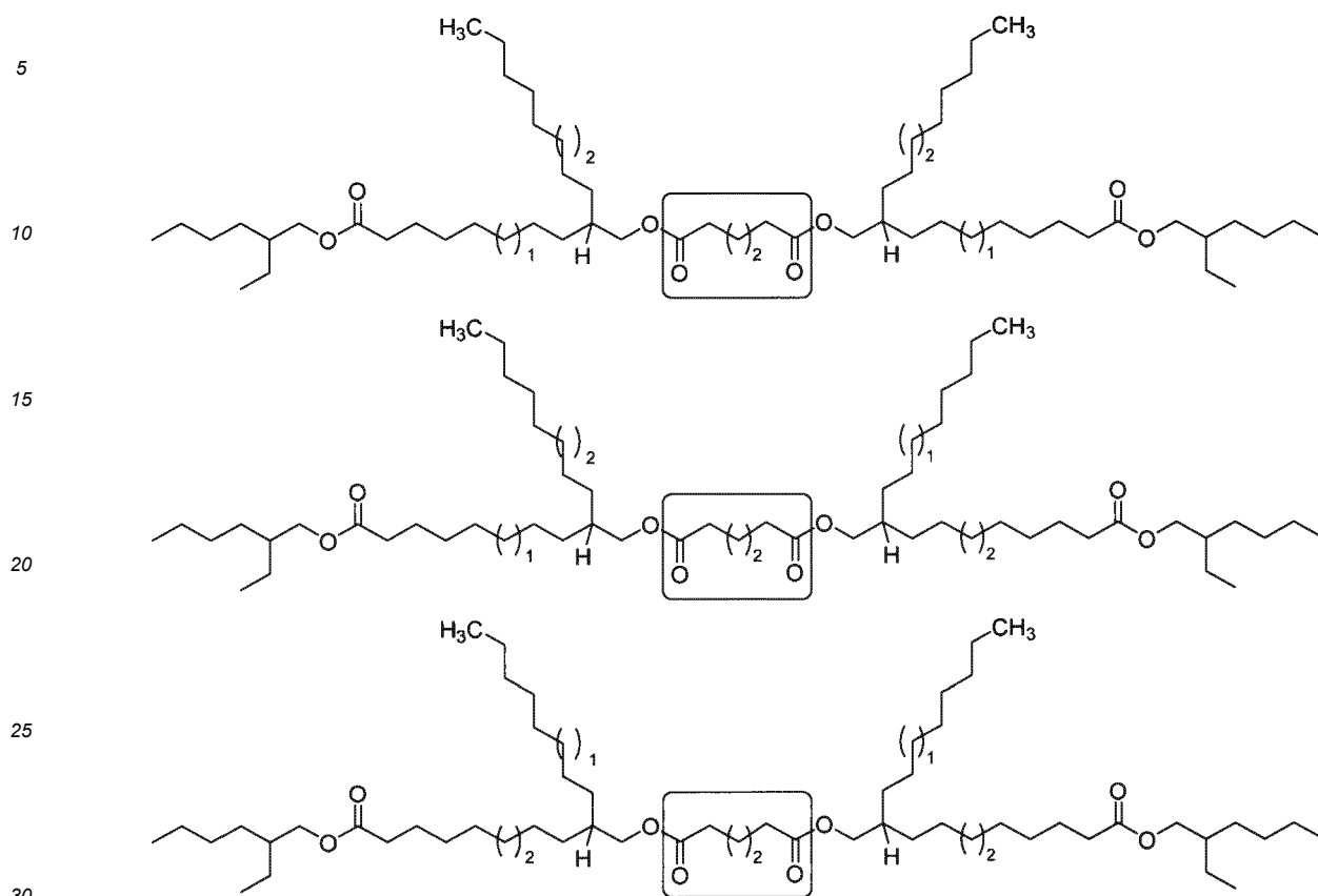
Abbildung 8. Besonders bevorzugter Vertreter der erfindungsgemäßen Verbindungen gemäß der bevorzugten allgemeinen Struktur (Ic), hergestellt ausgehend von n -Hexandicarbonsäure als Dicarbonsäure-Komponente
