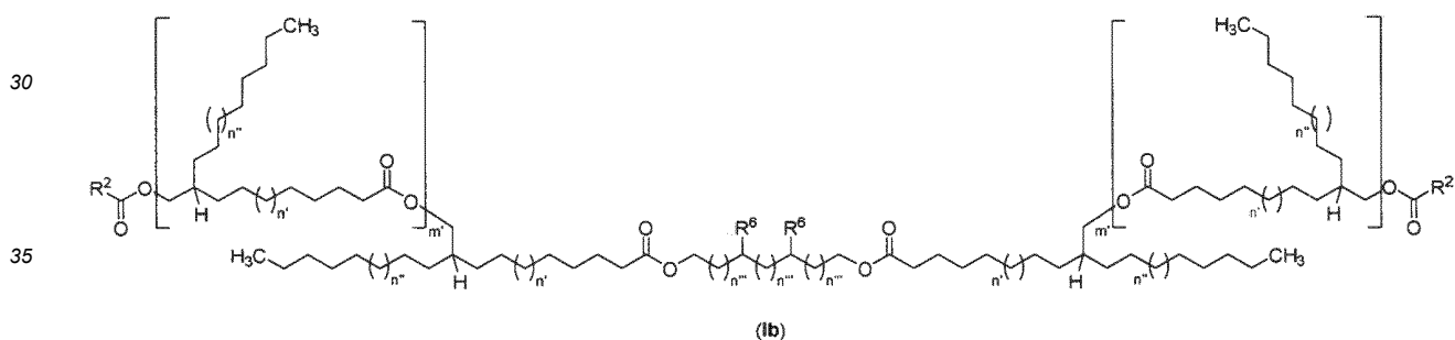
Abbildung 3. Besonders bevorzugte Vertreter der erfindungsgemäßen Verbindungen am Beispiel der Ölsäurederivate (Ib)
