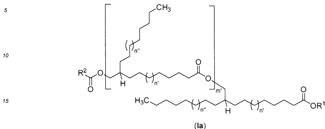
20 Abbildung 2. Besonders bevorzugte Vertreter der erfindungsgemäßen Verbindungen am Beispiel der Ölsäurederivate (Ia)
