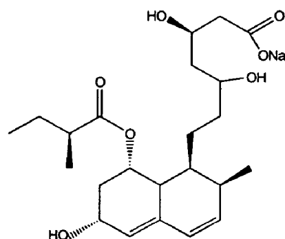
59-0329 (hydrolyzed pravastatin)
