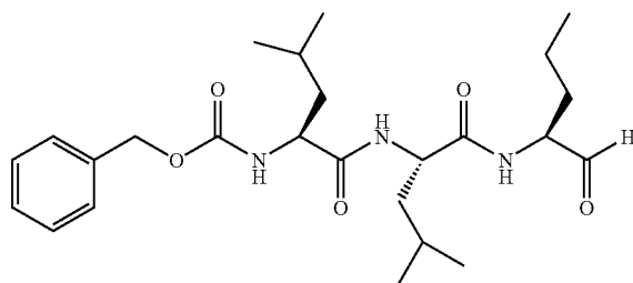
Z-Leu-Leu-Nva-CHO
