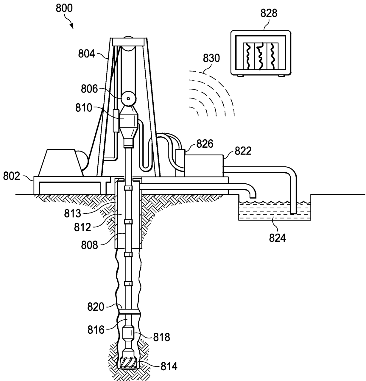
FIG. 8A
