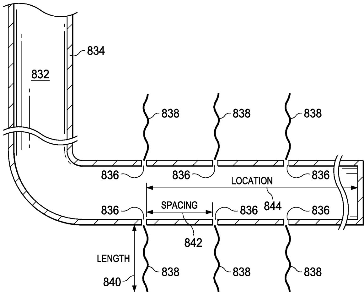
FIG. 8B
