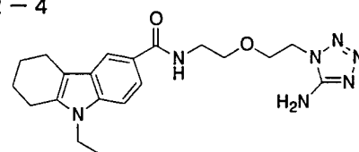
化合物 2-4
