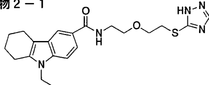
化合物 2-1
