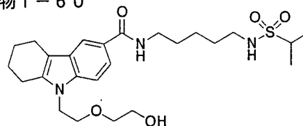
化合物 1-60
