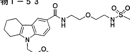
化合物 1-53
