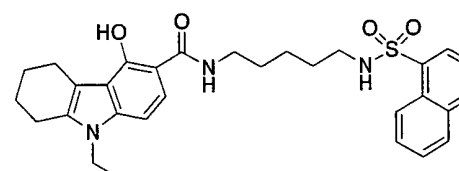
化合物 1-44
