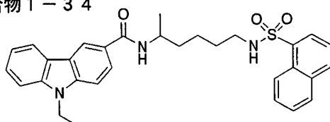
化合物 1-35
