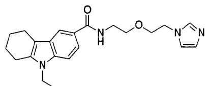
化合物 2-3
