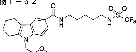
化合物 1-62
