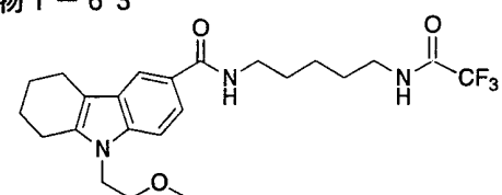
化合物 1-63
