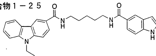
化合物 1-26
