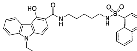
化合物 1-42
