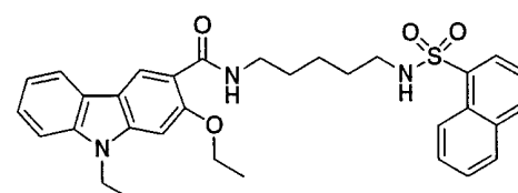
化合物 1-39
