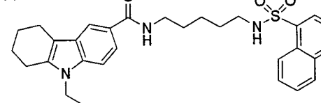
化合物 1-46
