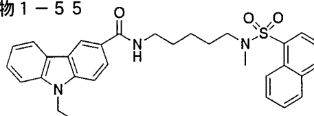
化合物 1-55
