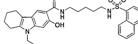
化合物 1-44
