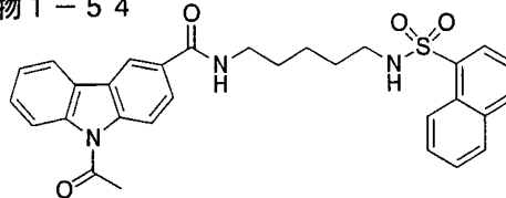
化合物 1-54
