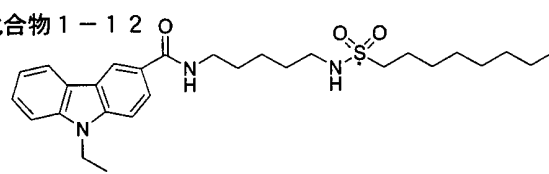
化合物 1-13
