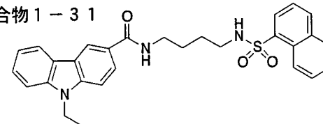
化合物 1-32
