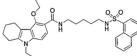
化合物 1-41
