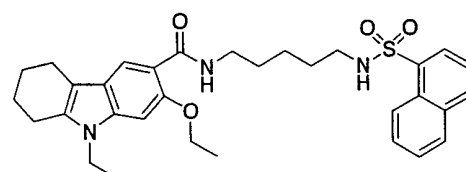
化合物 1-38
