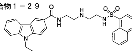
化合物 1-30
