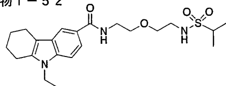
化合物 1-52
