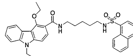
化合物 1-39
