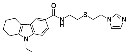
化合物 2-2
