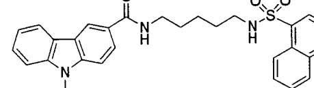
化合物 1-46
