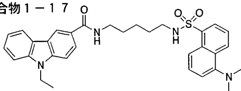
化合物 1-18
