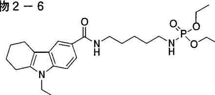
化合物 2-6
