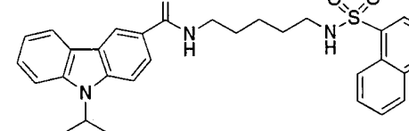
化合物 1-47
