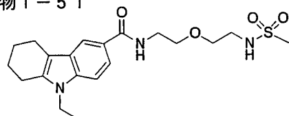
化合物 1-51
