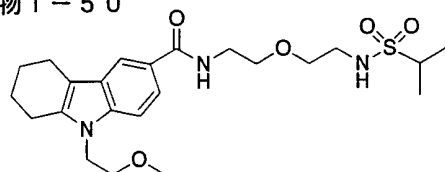
化合物 1-50
