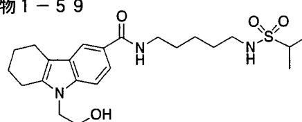
化合物 1-59
