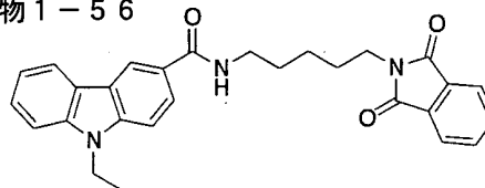
化合物 1-56
