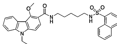
化合物 1-37
