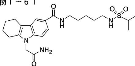
化合物 1-61
