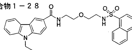
化合物 1-29
