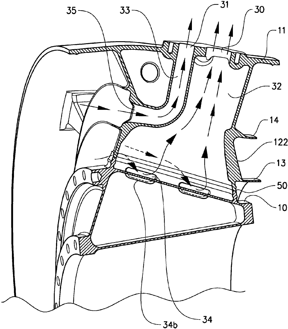
FIG. 5 BB
