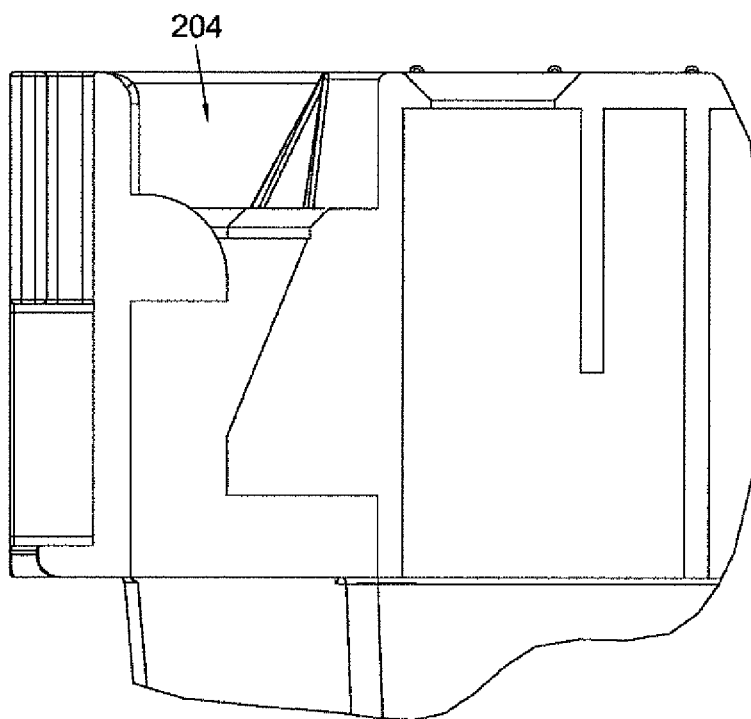
Fig. 74 SECTION D-D
