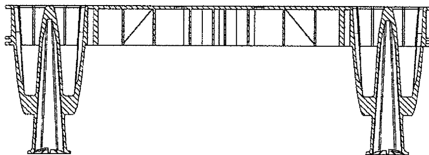
Fig. 80 Section A-A
