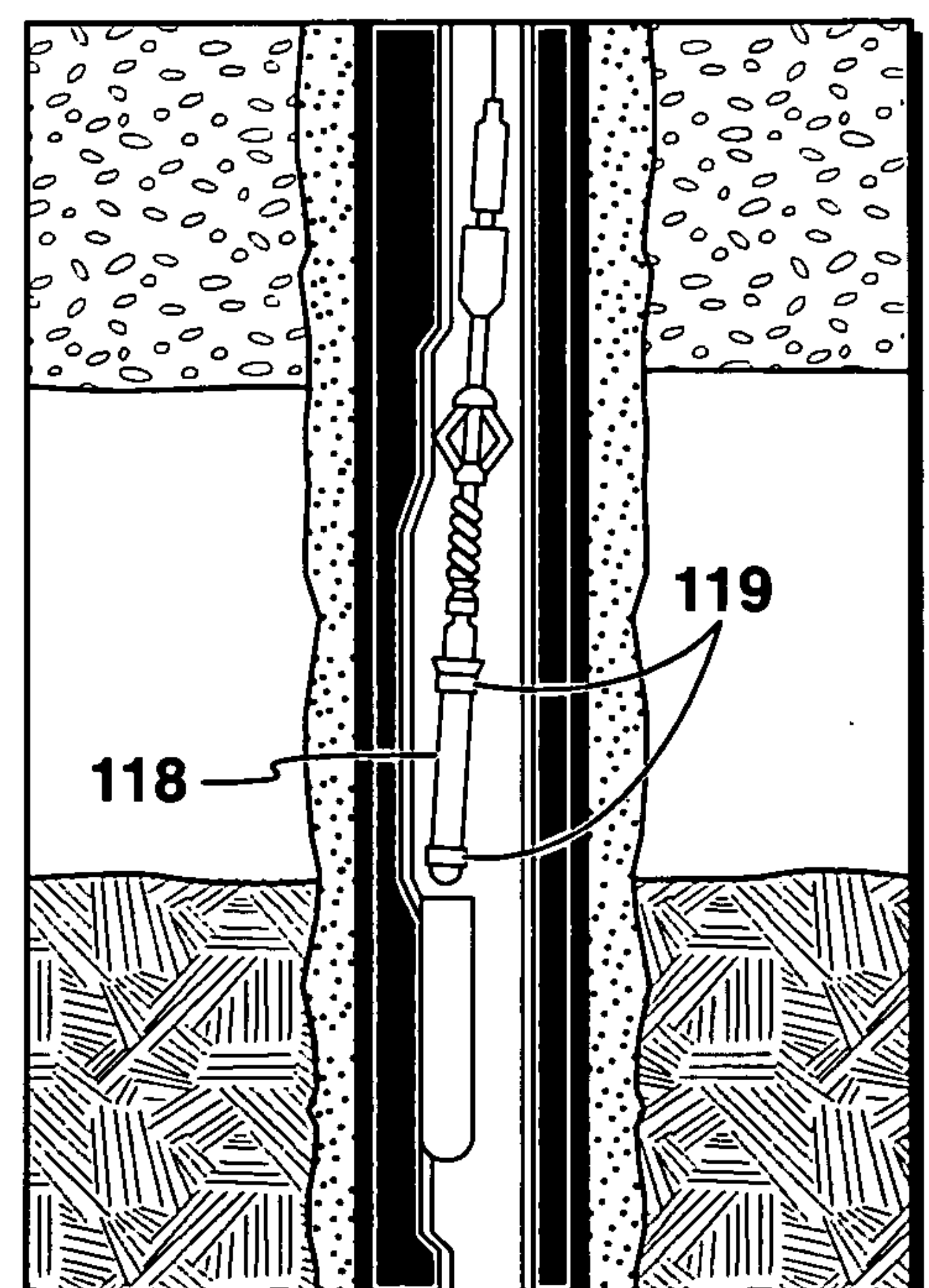
FIG. 9E
