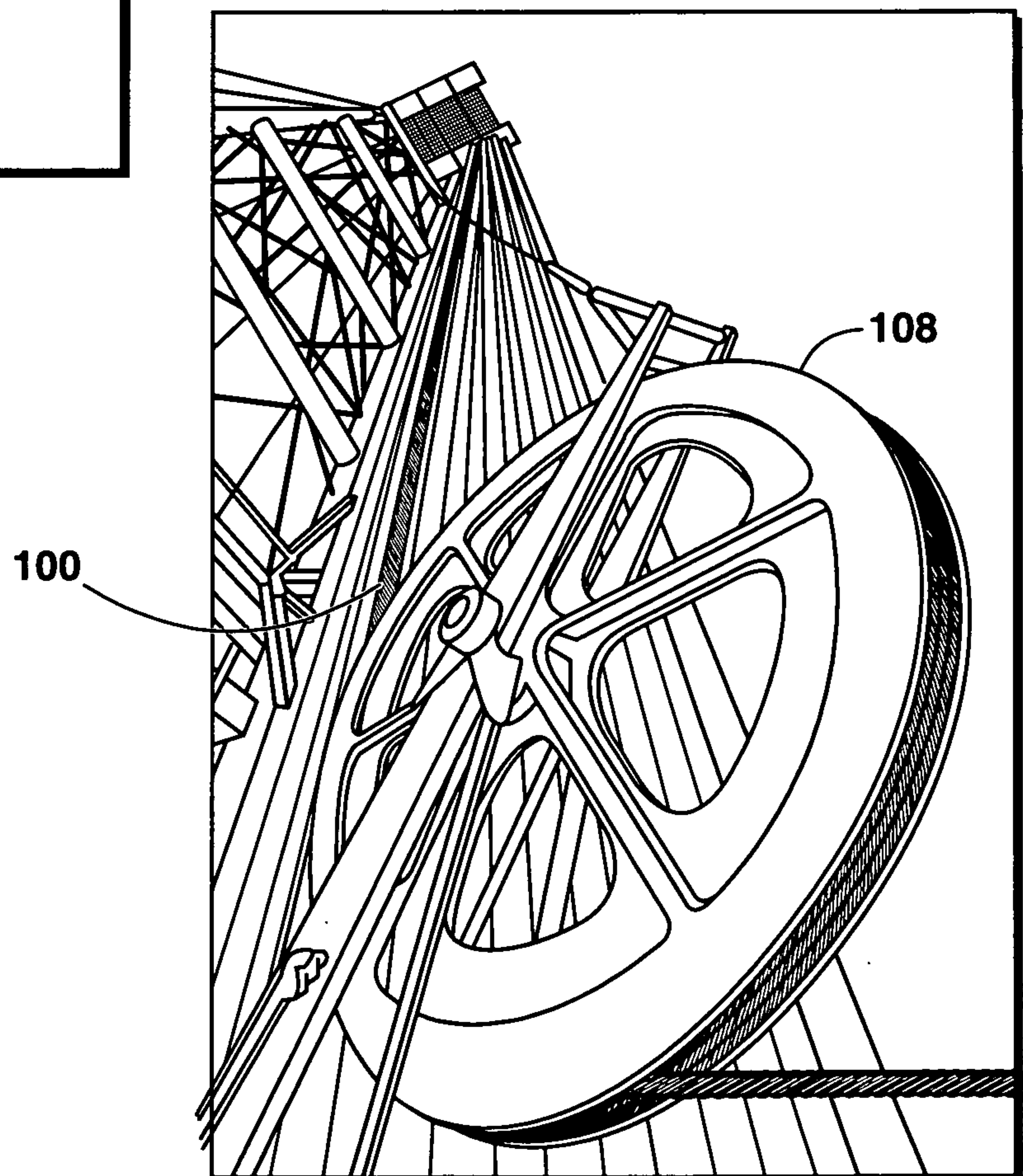
FIG. 7B
