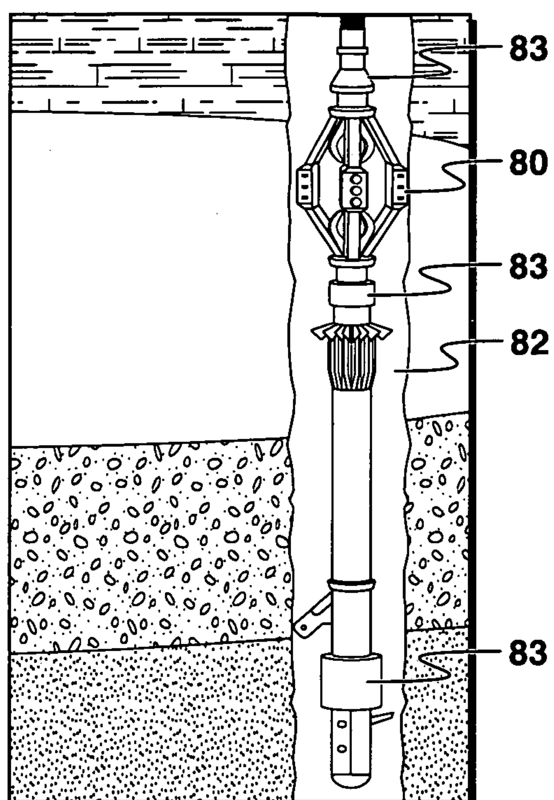
FIG. 6A
