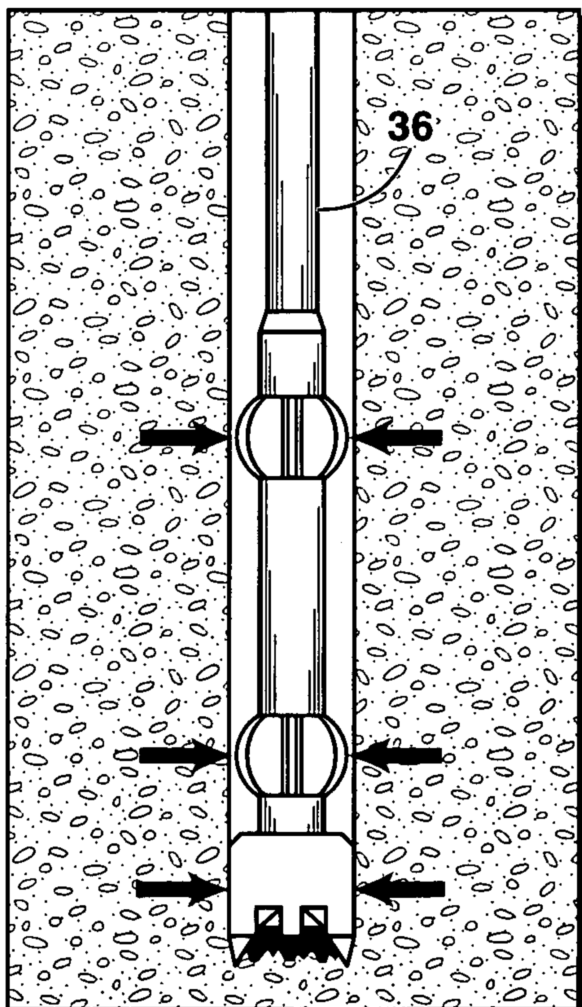
FIG. 2C
