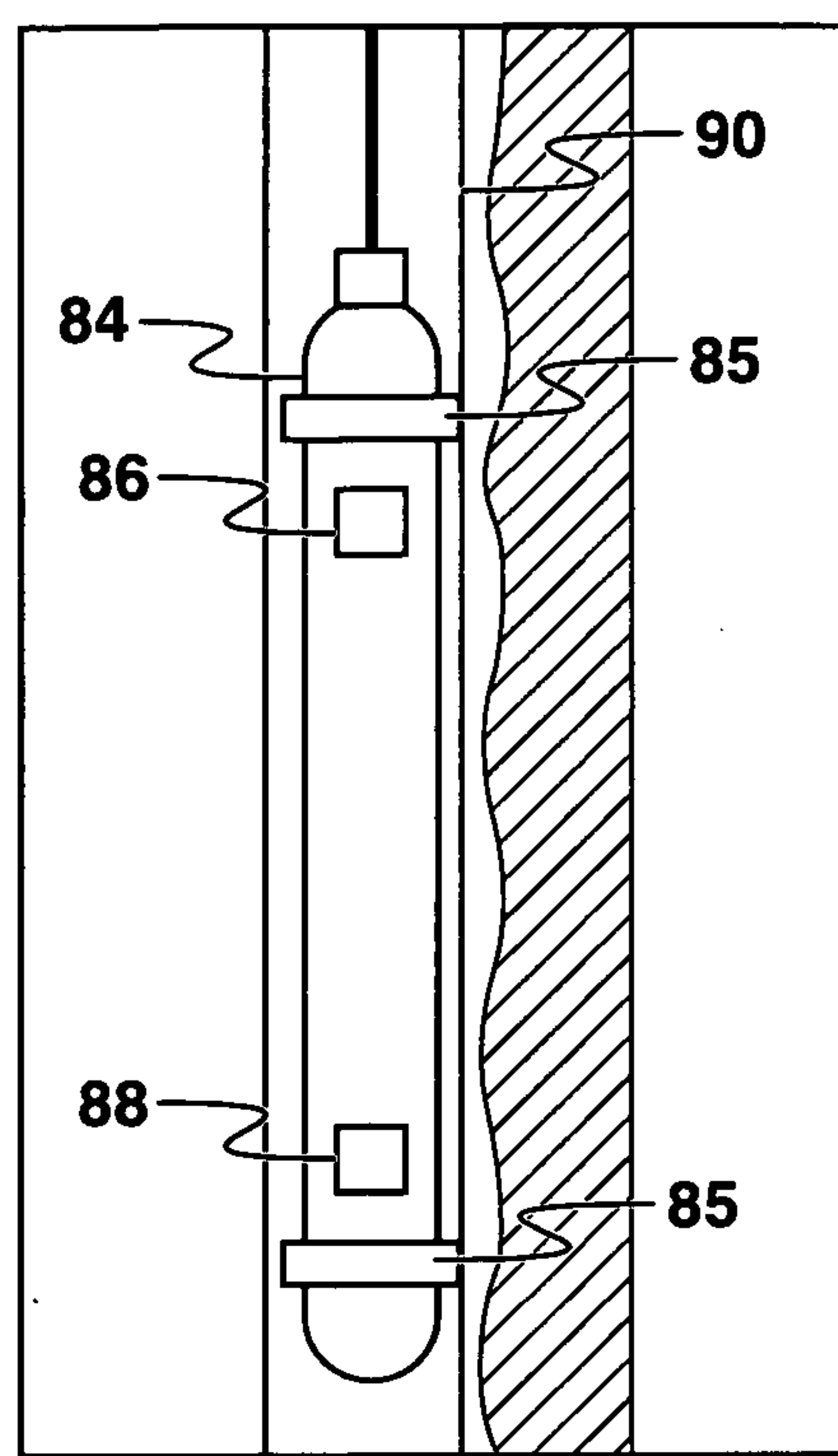
FIG. 6B
