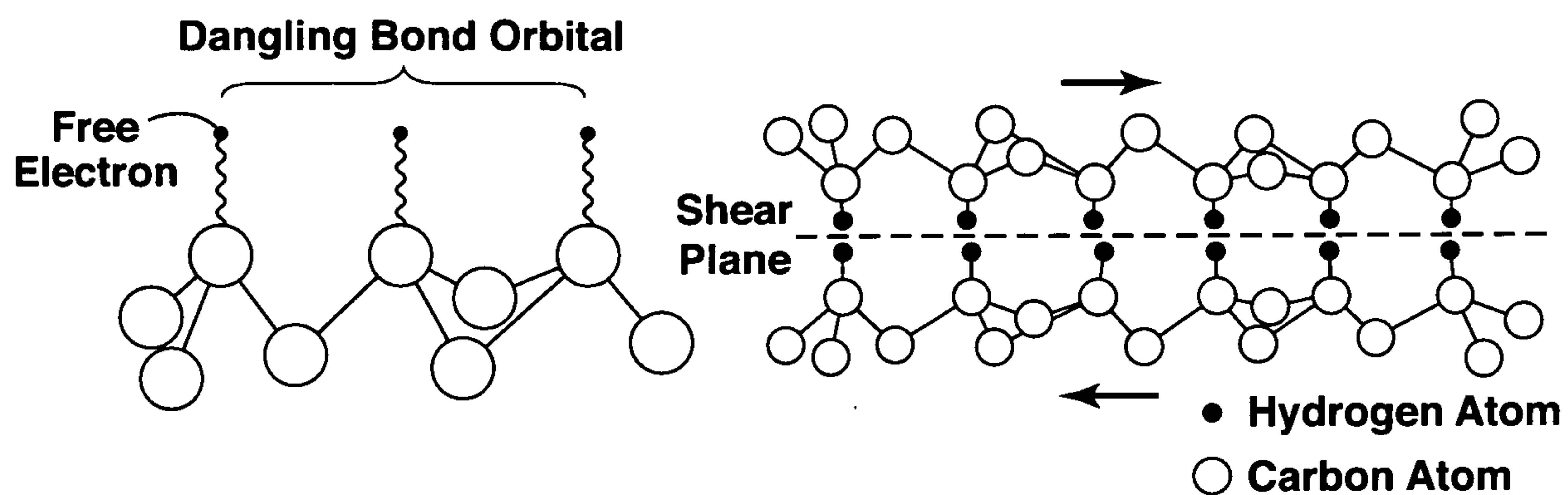
FIG. 18
