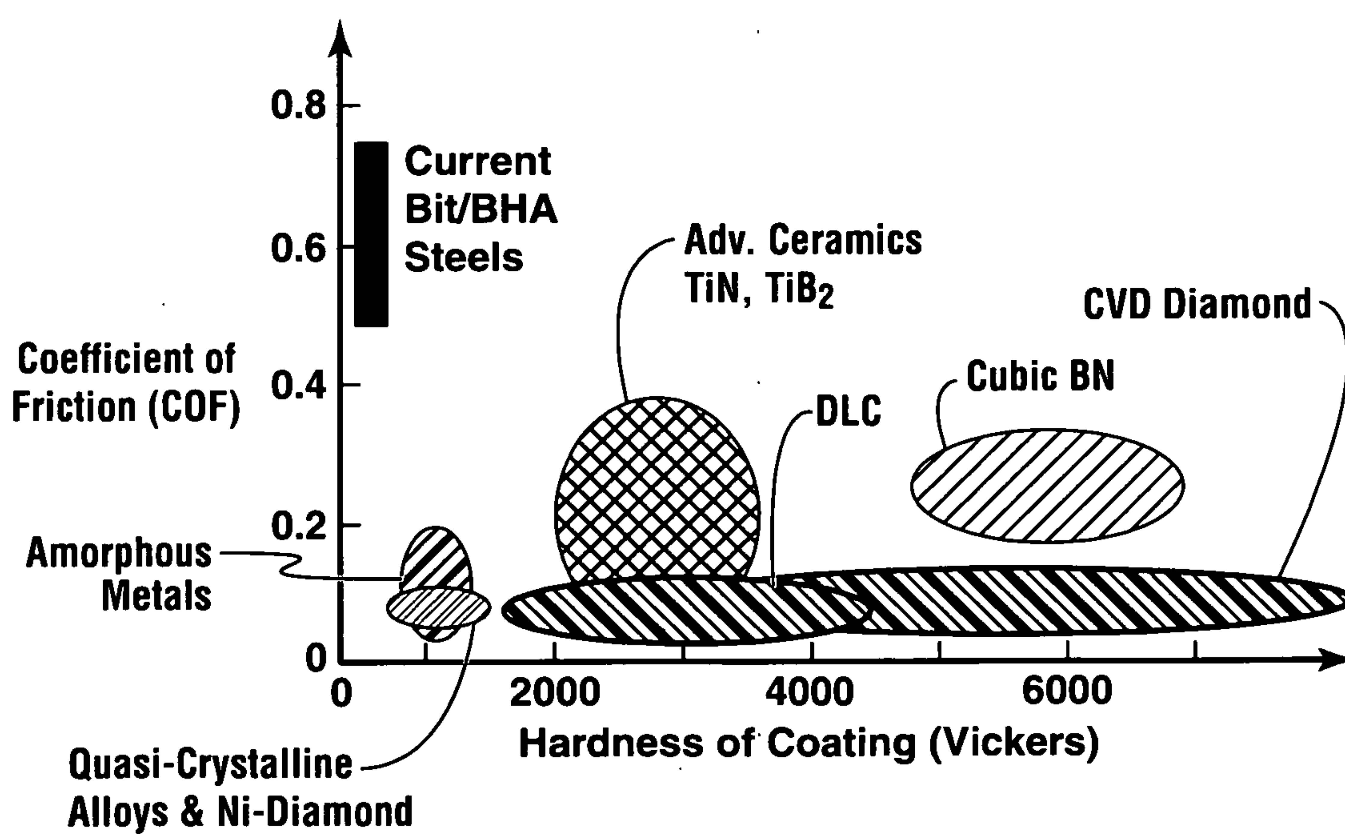
FIG. 15
