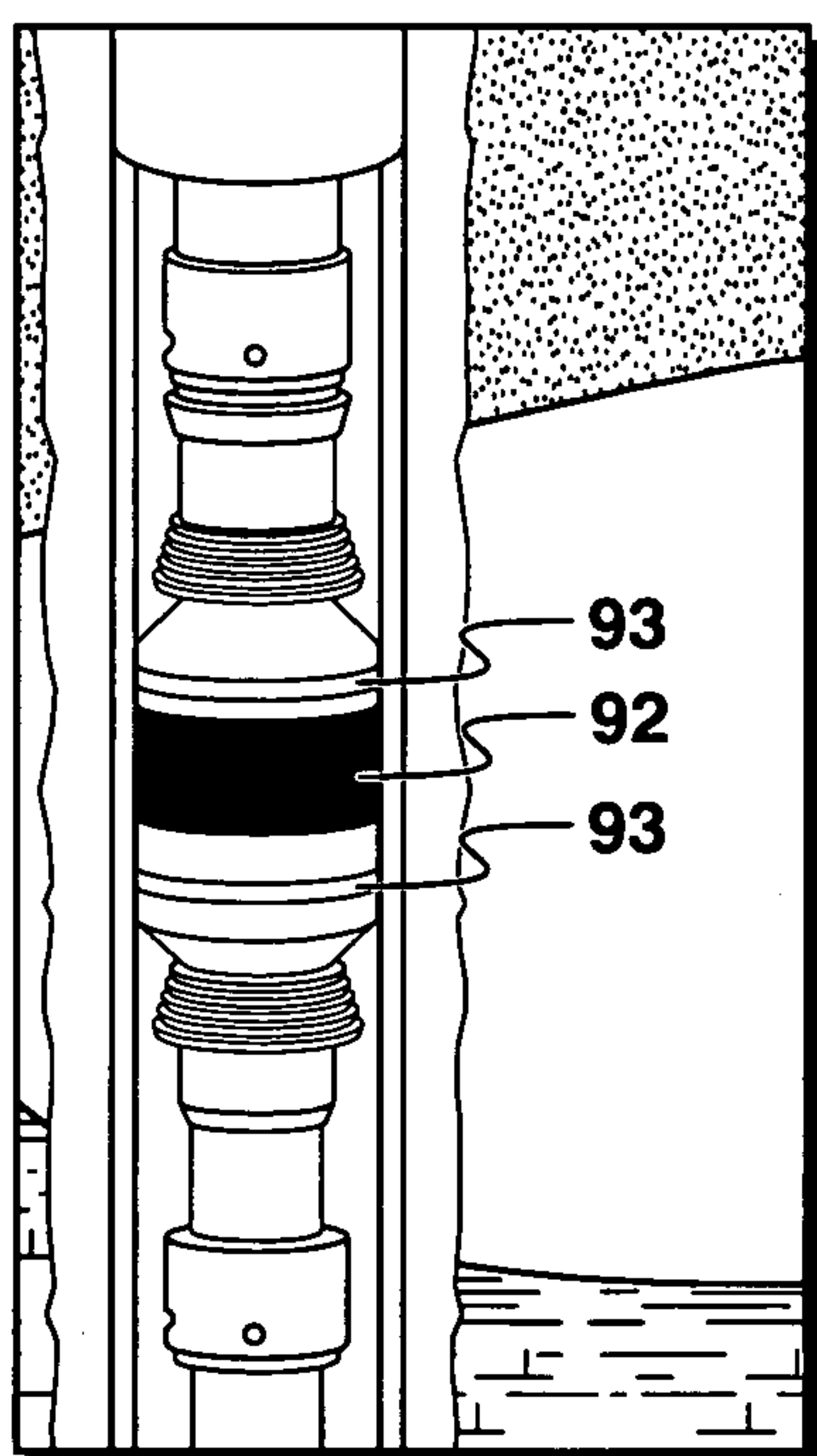
FIG. 6C
