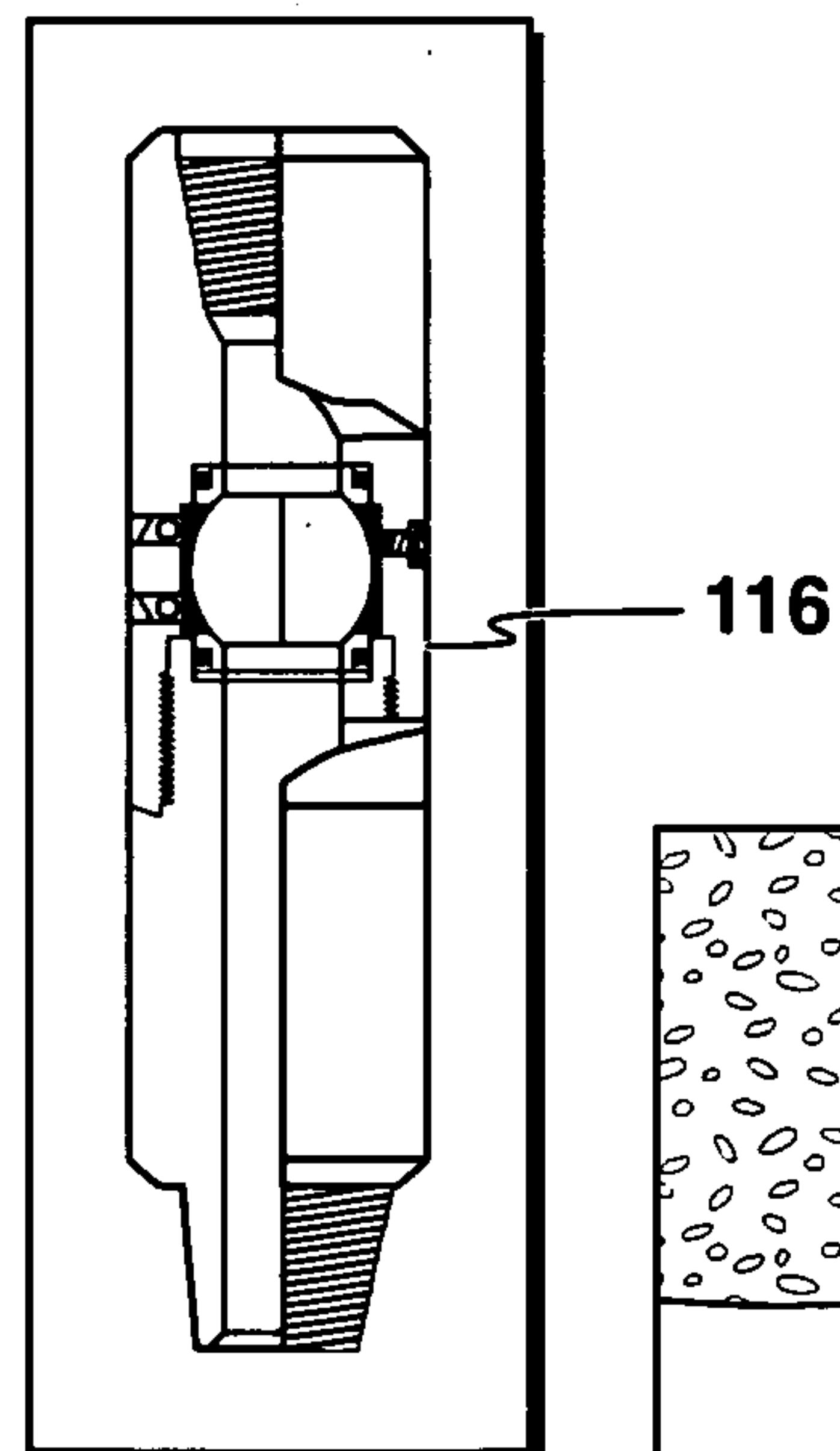
FIG. 9D
