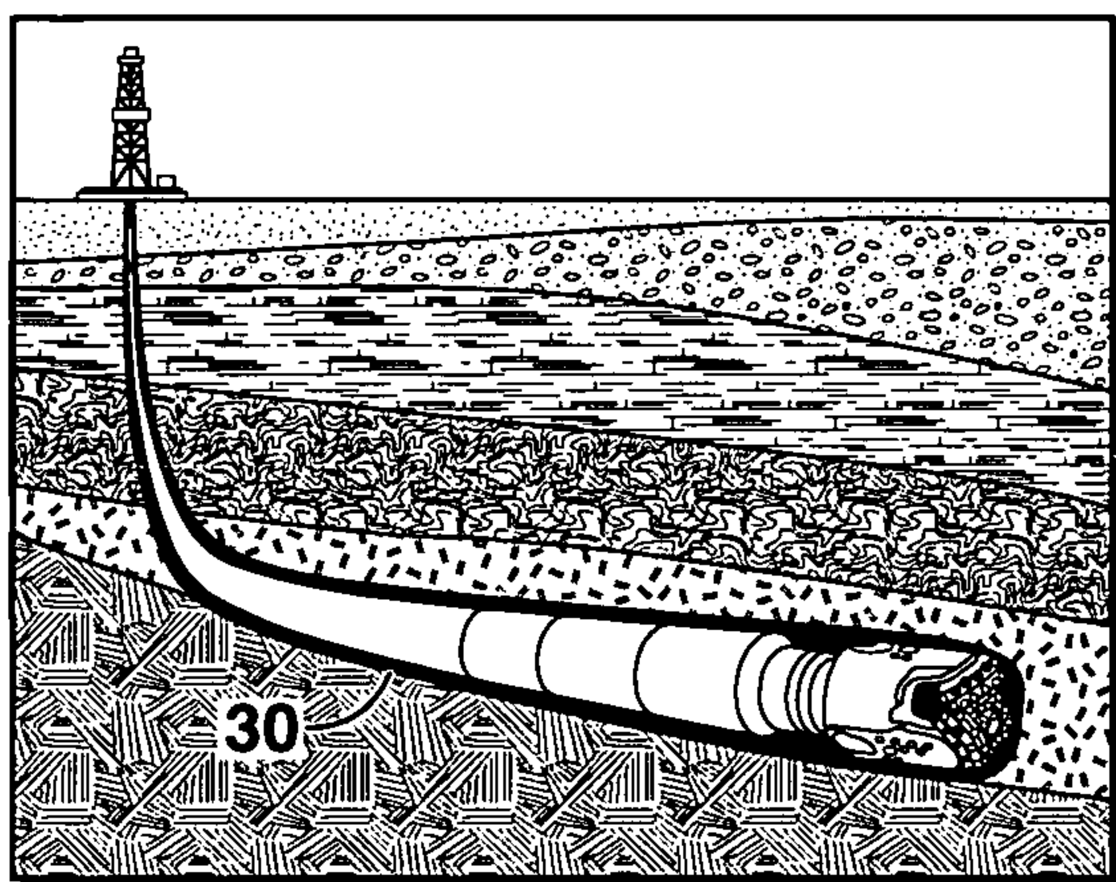
FIG. 2A
