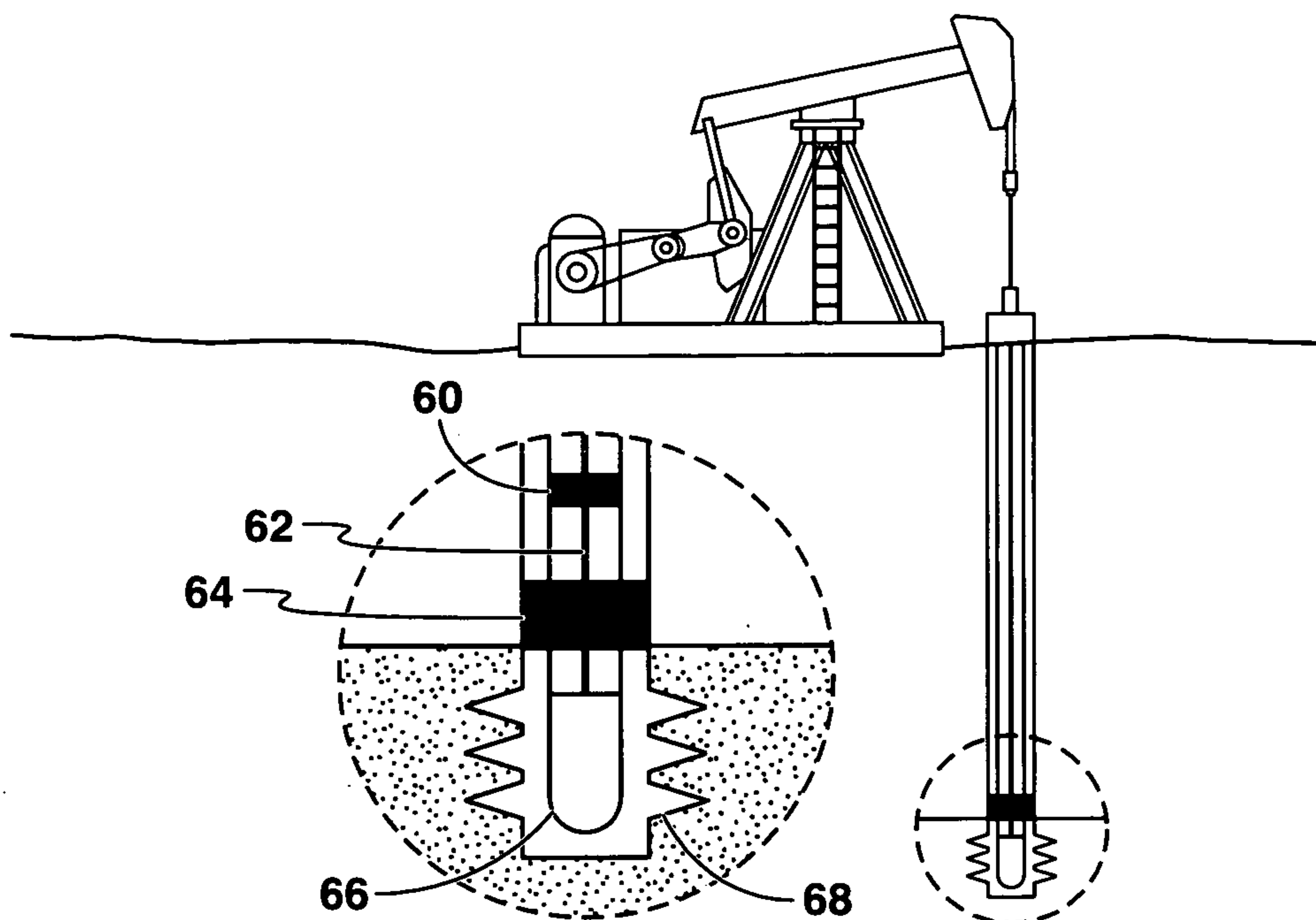
FIG. 5A
