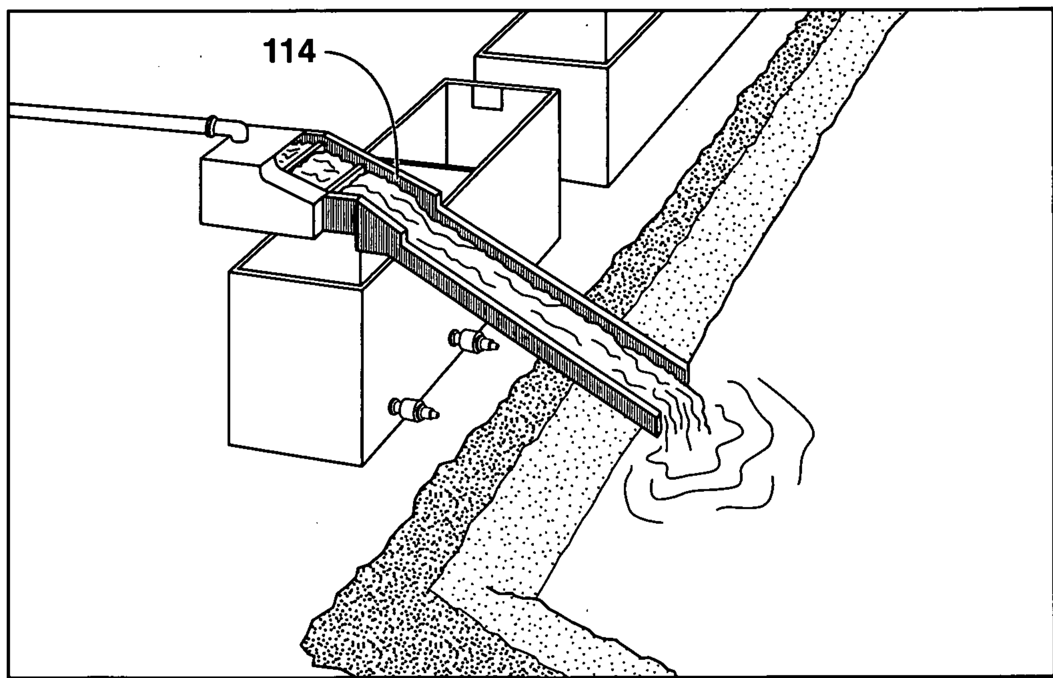
FIG. 8C
