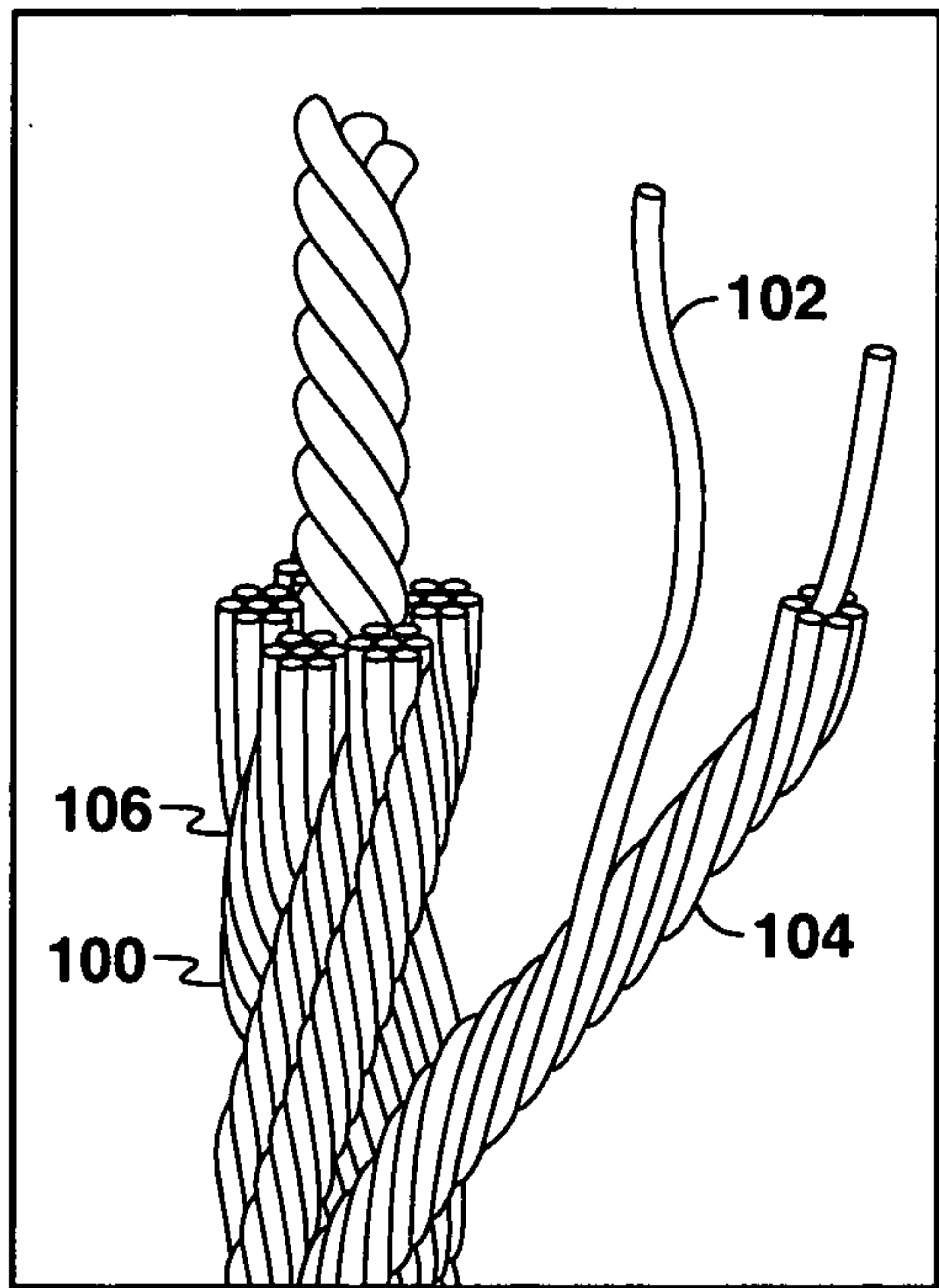
FIG. 7A
