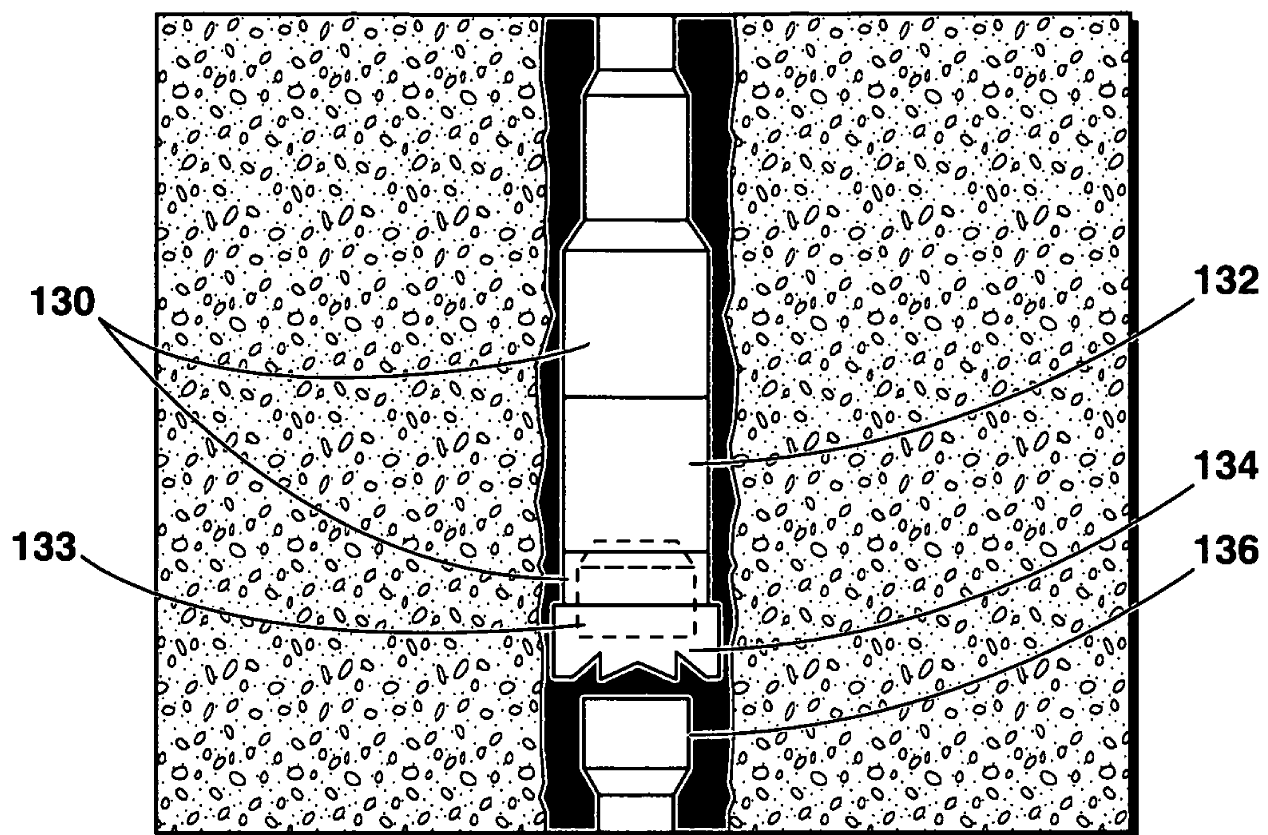
FIG. 11A
