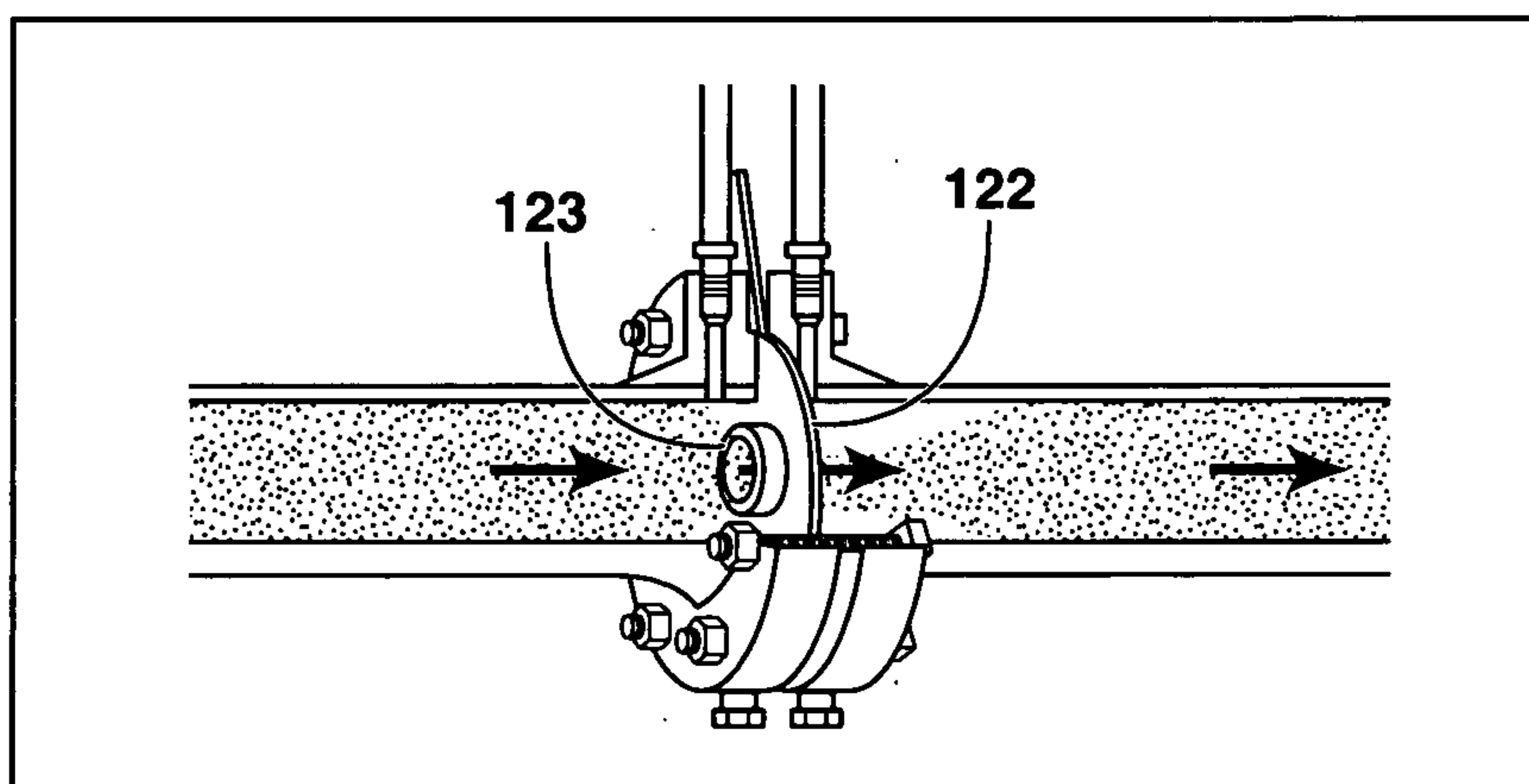
FIG. 10B
