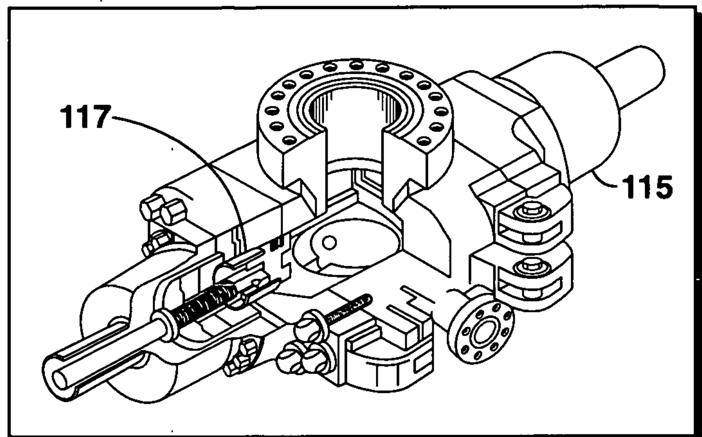
FIG. 9B
