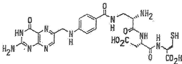
EC31 (Pte-L-βDpr-L-Asp-L-Cys)
