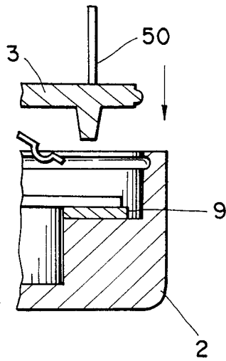
FIG. 9 A
