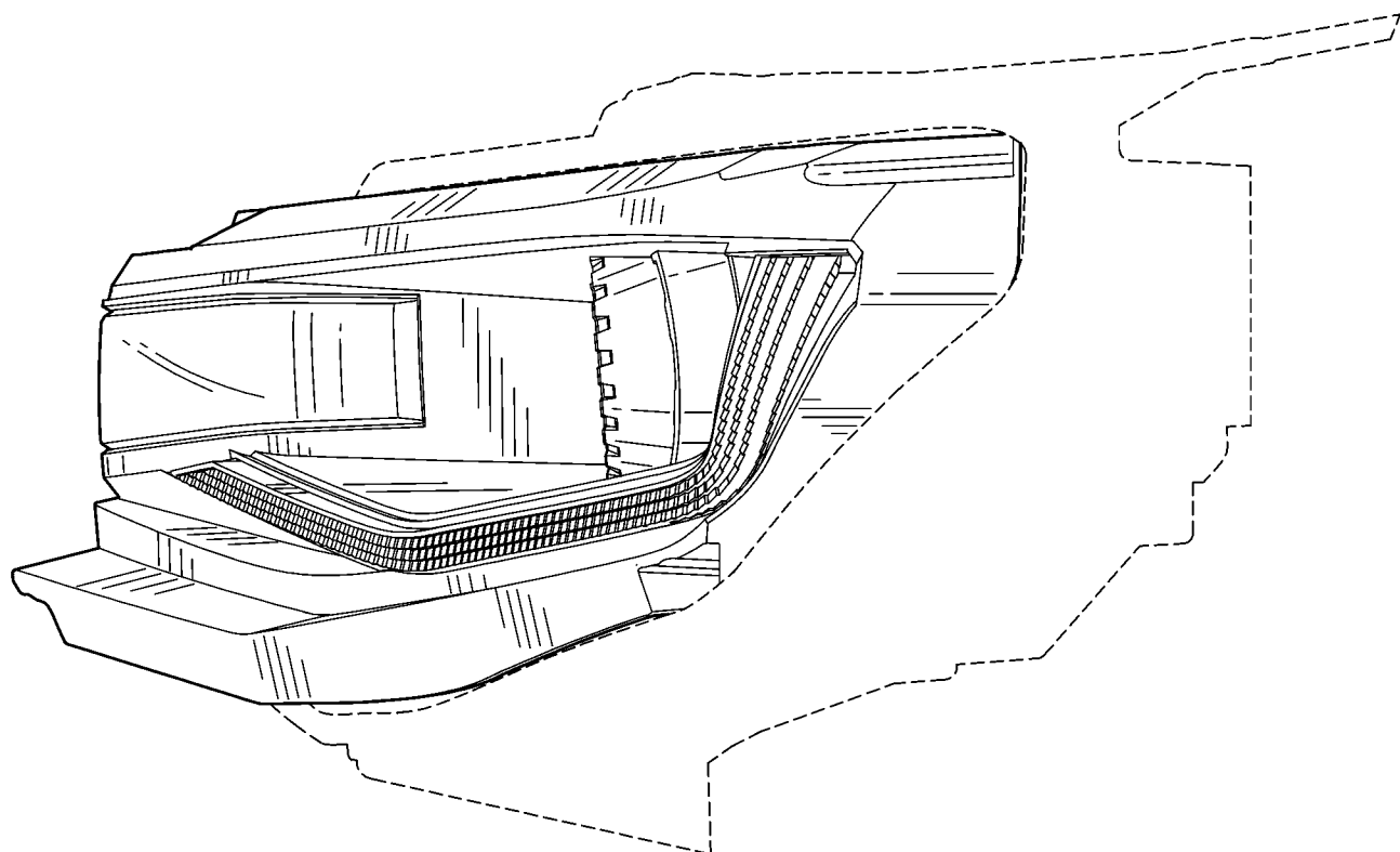
右側視圖
