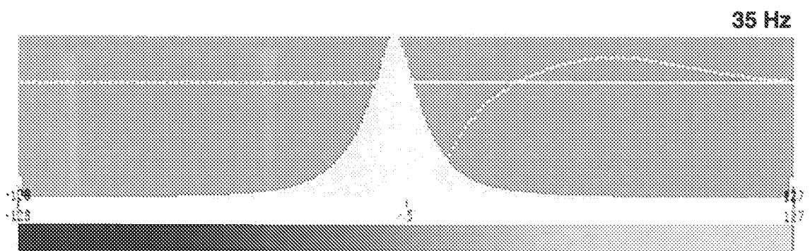
FIG. 10B
