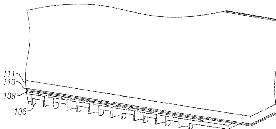
FIG. 18C
