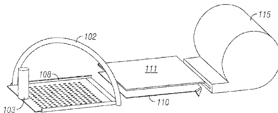
FIG. 18D
