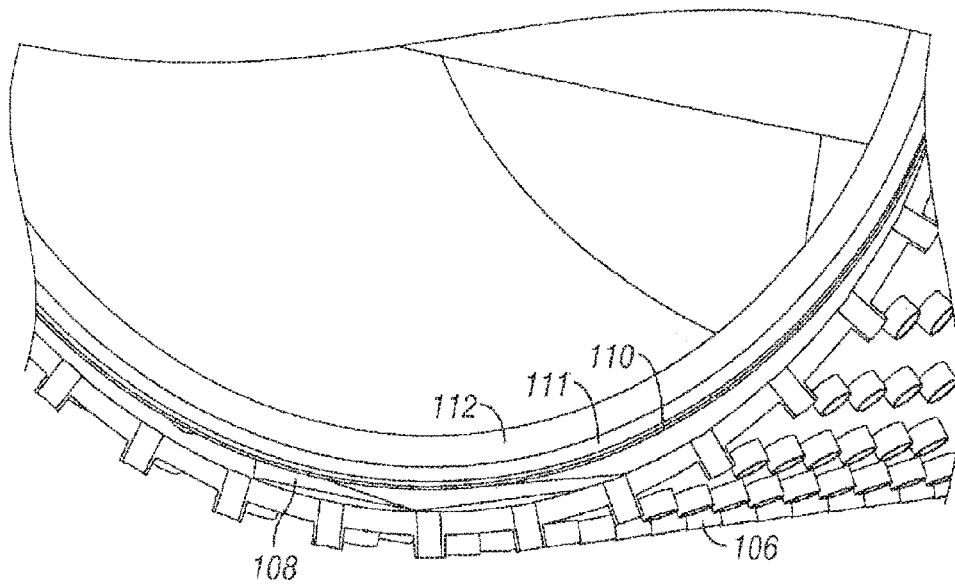
FIG. 14C
