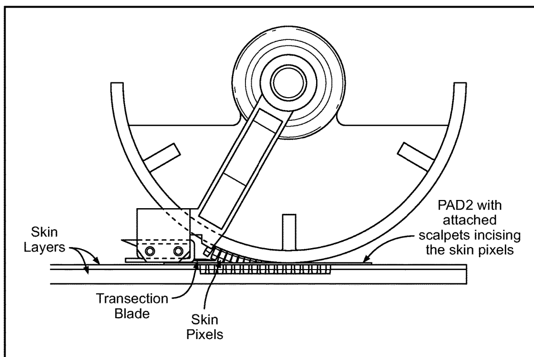
FIG. 13E
