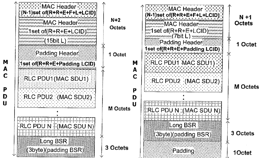
(b) case 2, implicit padding BSR
