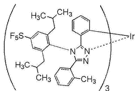
[\text{Ir}(\text{mpptz}-\text{diBuSF}_5\text{p})_3]
