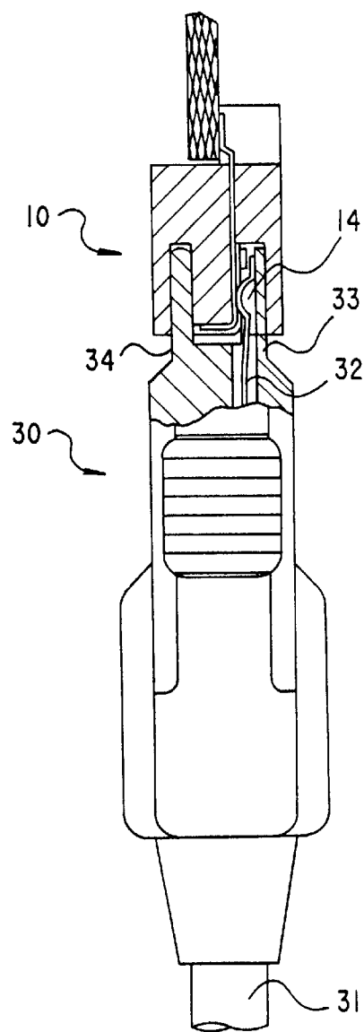
FIG.2B
