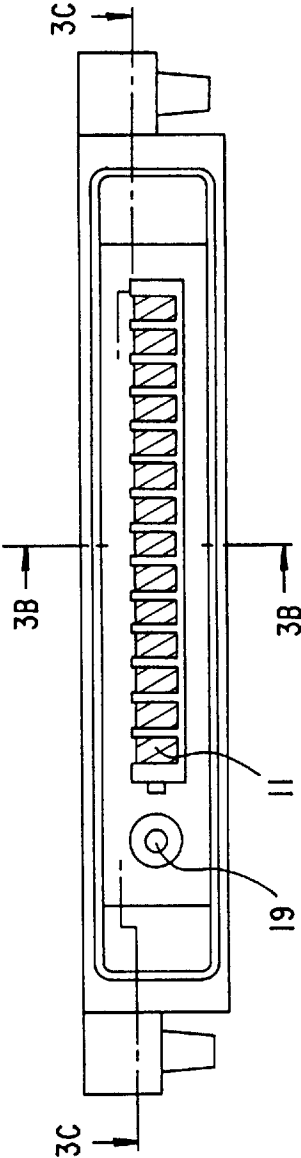
FIG.3A
