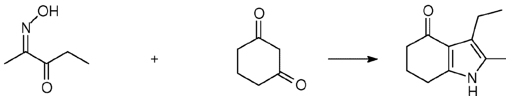
2,3-Pentanedione-2-oxime (SUMO-1) 1,3-Cyclohexanedione
