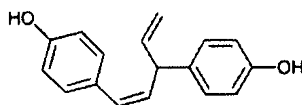
Nyasol
