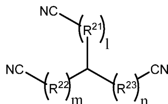
Formule II-A,
