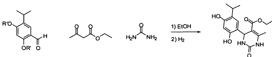
5 Scheme III:
