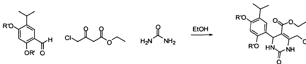
5 Scheme III:
