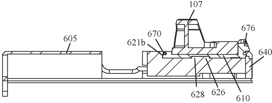
FIG. 7B SECTION A-A
