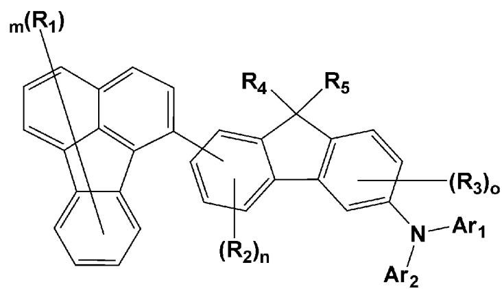
[화학식 10]
