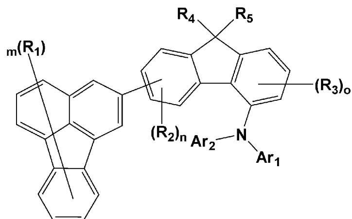
[화학식 8]
