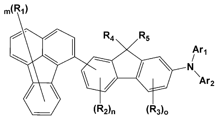
[화학식 9]
