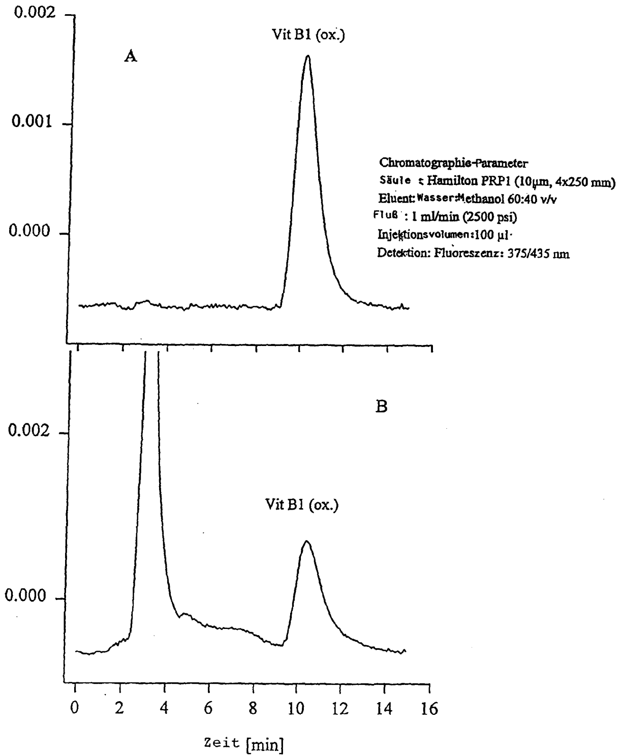
Chromatogramme einer Standardlösung (104 µg/g Thiaminhydrochlorid) und der Probe B056 (Bockshornkleekeimlinge nach 3 Tagen Keimzeit)
