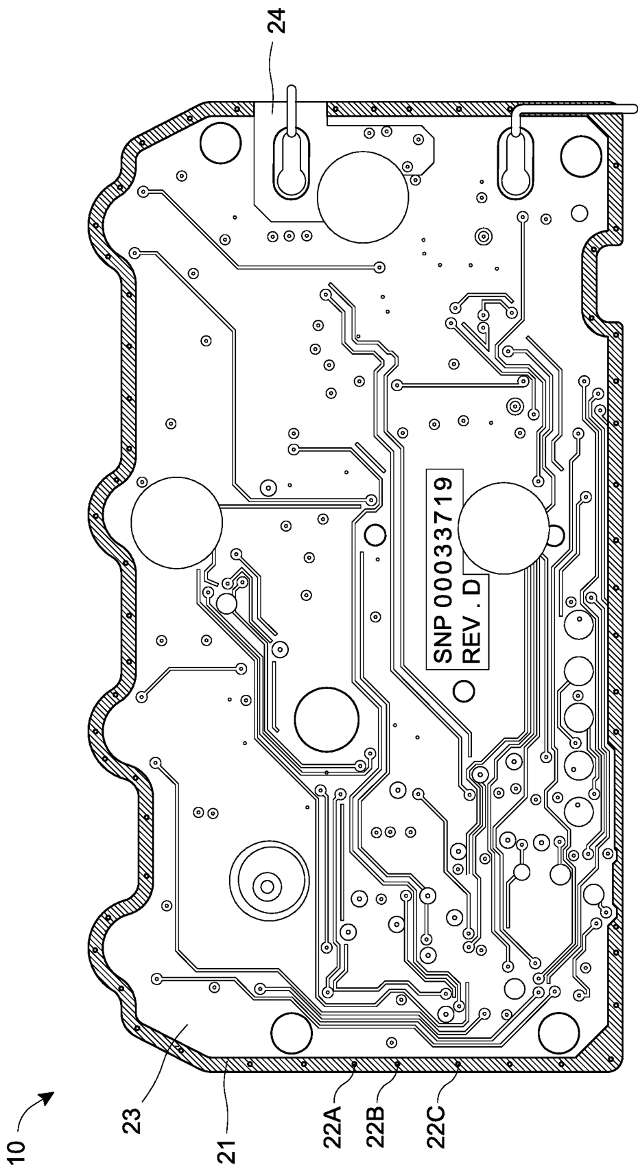
FIG. 20B
