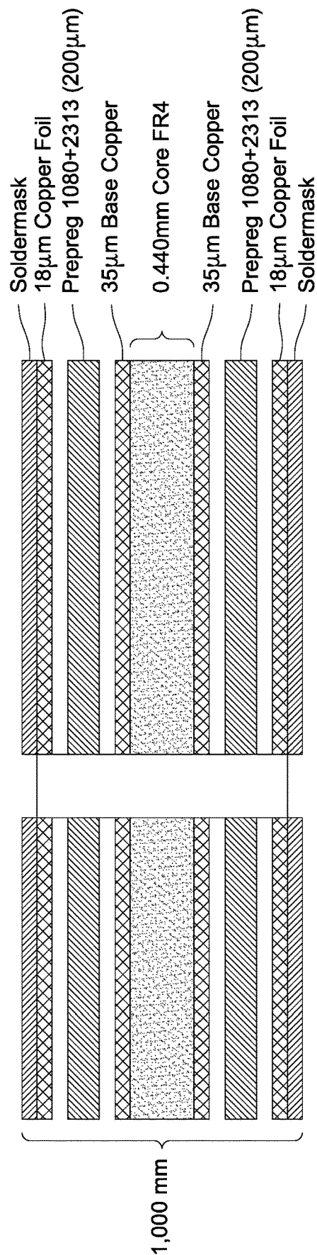
FIG. 24
