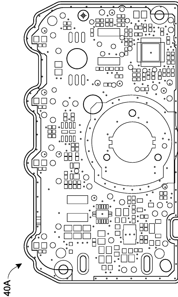
FIG. 22A
