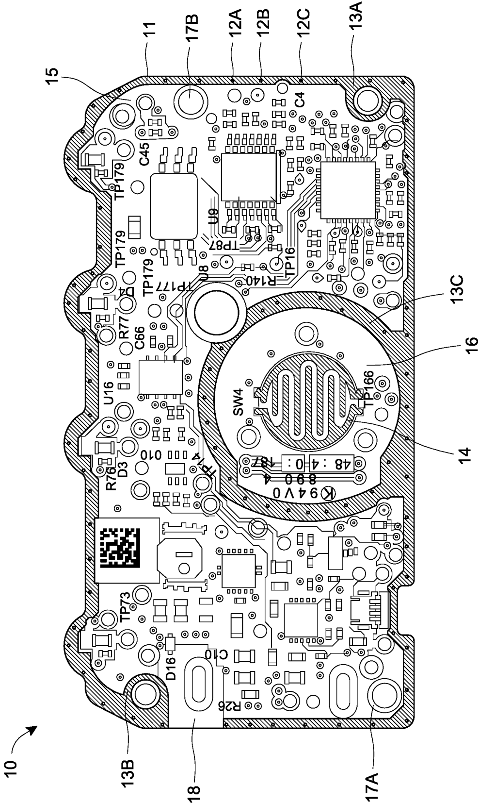
FIG. 20A
