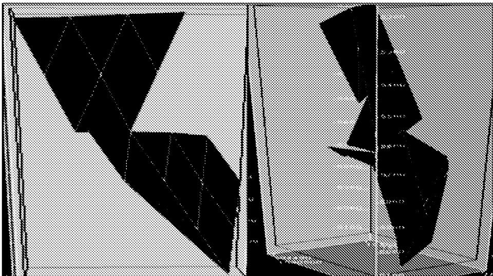
FIG. 3F
