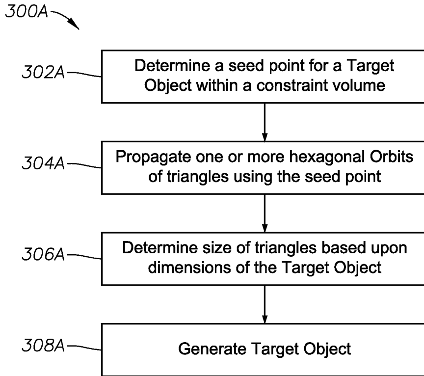
FIG. 3I
