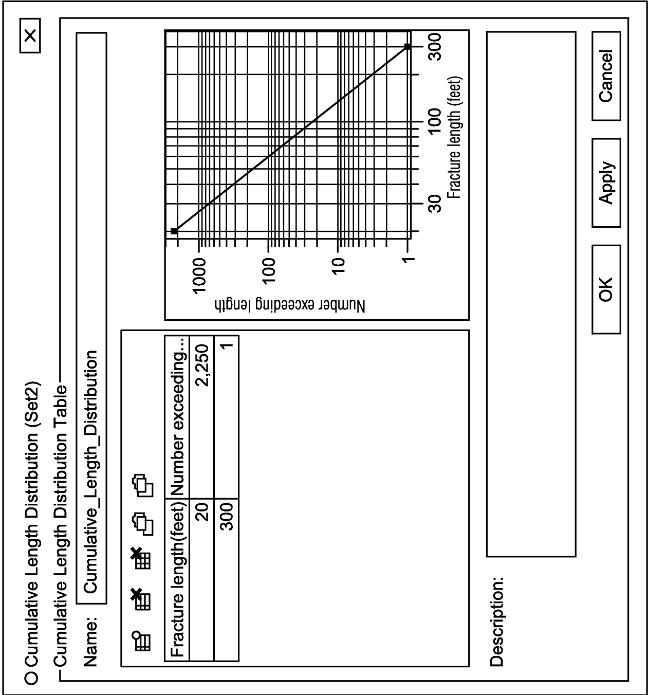
FIG. 4I
