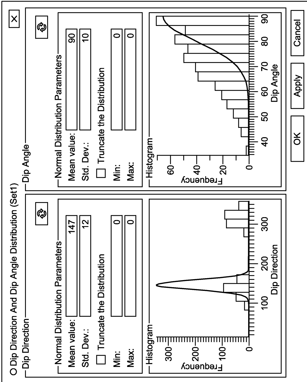
FIG. 4D
