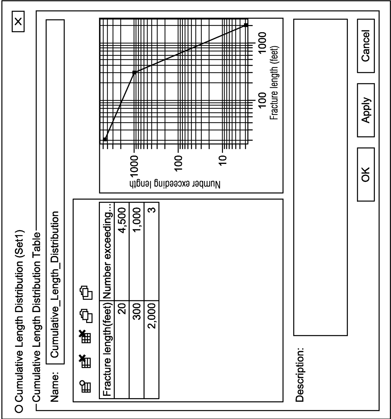
FIG. 4F
