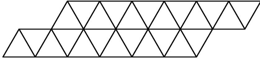
FIG. 3G
