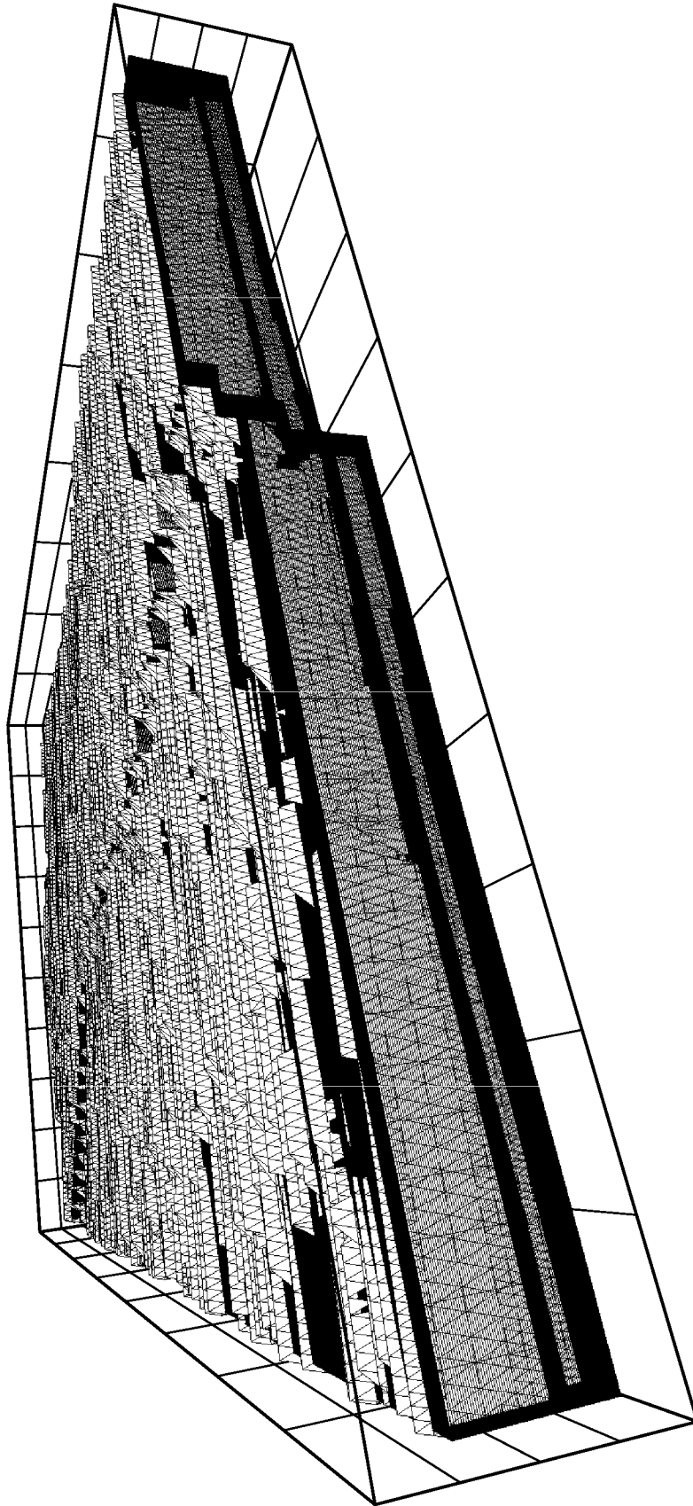
FIG. 5D
