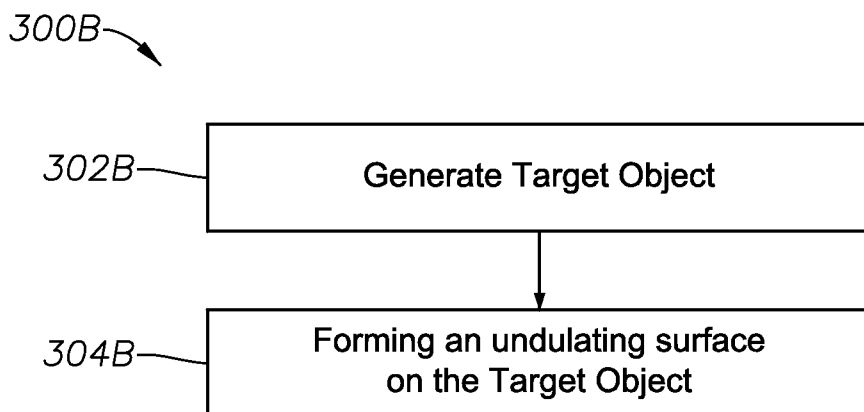
FIG. 3J
