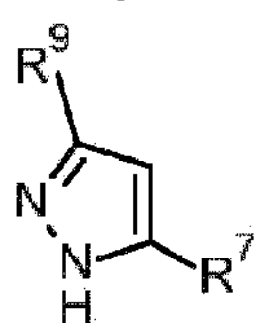
1H tautomer
