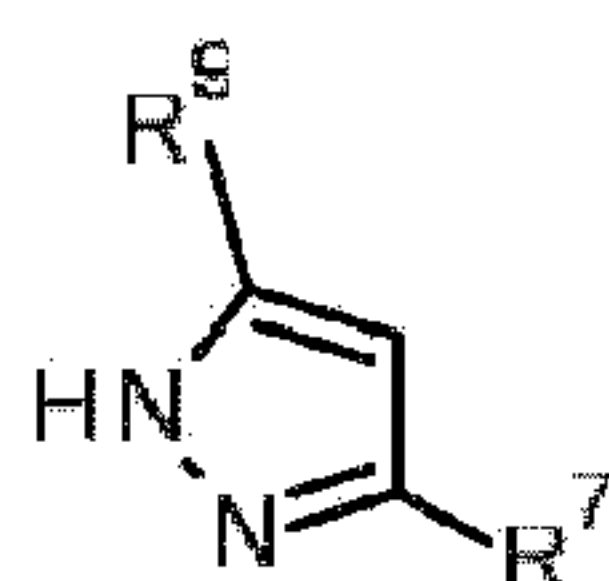
2H tautomer
