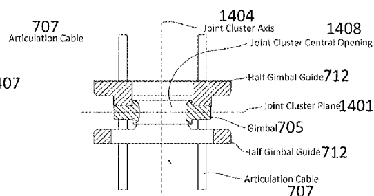
SECTION A-A FIG. 14C
