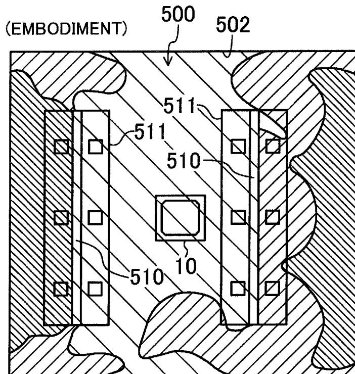
FIG.10B
