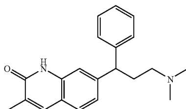
Co. No. 3; Ex. [B3]
