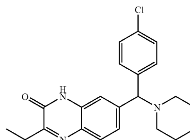
Co. No. 5; Ex. [B5]
