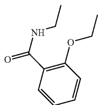
2ETHOXYBENZAMIDENETHYL
