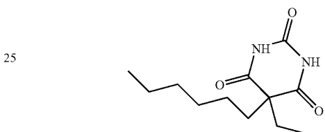
BARBITURICACID5HEXYL5ETHYL
