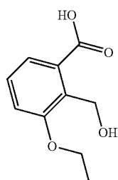
BENZOICACID2HYDROXYMETHYL3ETHOXY
