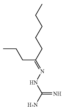
4NONANONEGUANYLHYDRAZONE
