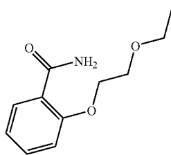
ETOSALAMIDE
