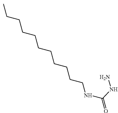
4UNDECYLSSEMICARBAZIDE
