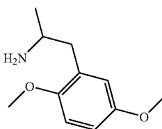
25DIMETHOXYAMPHETAMINE
