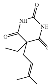
BARBITURICACID5ETHYL53METHYLBUTEN2YL
