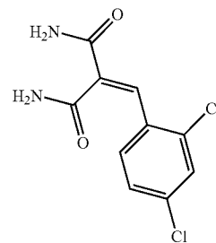
MALONAMIDE24DICHLOROENZAL
