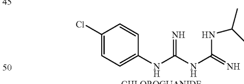
CHLOROGUANIDE
