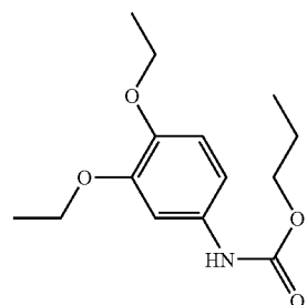
34DIETHOXYPHENYLCARBAMATEOPROPYL
