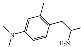
AMIFLAMINE
