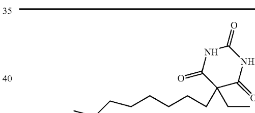
BARBITURICACID5OCTYL5ETHYL
