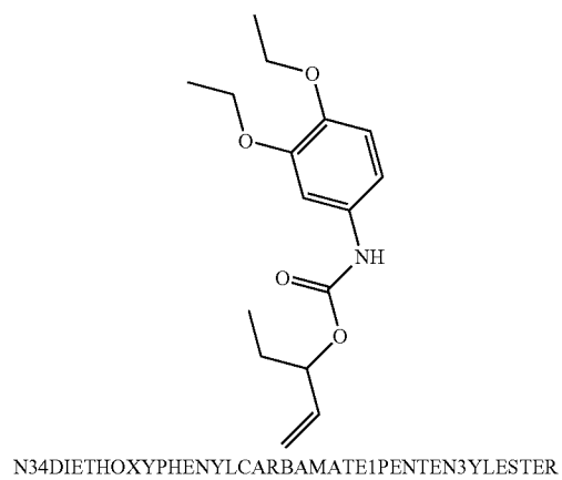
N34DIETHOXYPHENYLCARBAMATE1PENTEN3YLESTER
