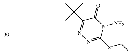
ETHIOZIN
