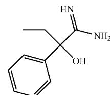
BENZENEMETHANOLAETHYLAAMIDINO
