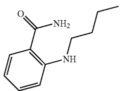
BENZAMIDEOBUTYLAMINO
