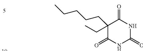
BARBITURICACID5AMYL5ETHYL
