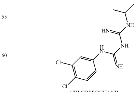
CHLORPROGUANIL
