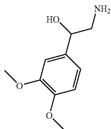
BENZENEETHANEAMINEHYDROXY34DIMETHOXY
