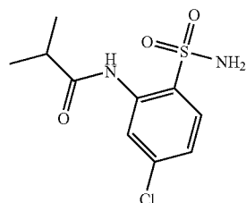
BENZENESULFONAMIDE2IBUTYROYLAMINO4CHLORO
