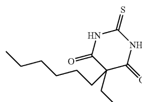
2THIO5ET5HEXYLBARBITURICACID
