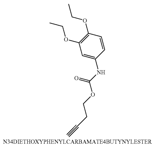
N34DIETHOXYPHENYLCARBAMATE4BUTYNYLESTER
