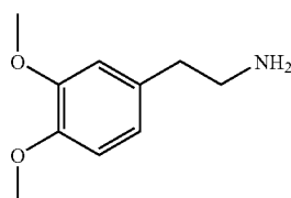
34DIMETHOXYPHENETHYLAMINE
