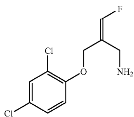
MDL72145
