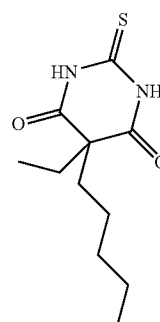
2THIO5ET5AMYLBARBITURICACID
