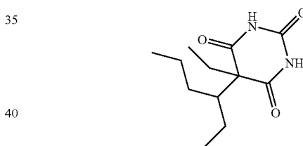
TETRABARBITAL
