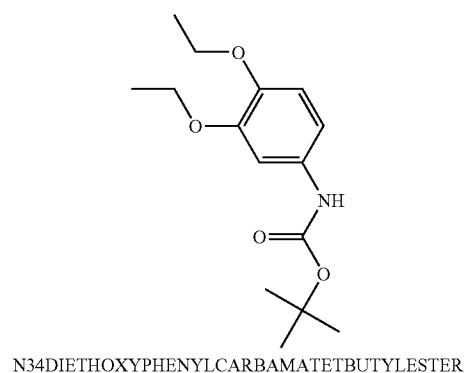
N34DIETHOXYPHENYLCARBAMATETBUTYLESTER
