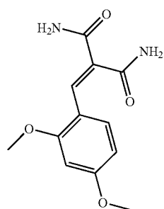
MALONAMIDE24DIMETHOXYBENZAL
