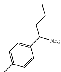
BUTYLAMINE1PTOLYL
