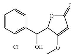
LOSIGAMONE
