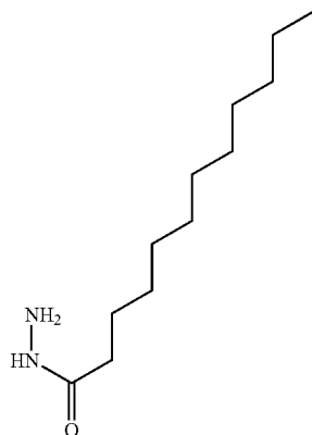
DODECANOICACIDHYDRAZIDE
