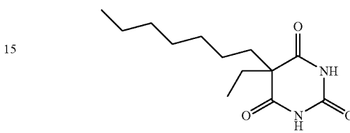
BARBITURICACID5HEPTYL5ETHYL
