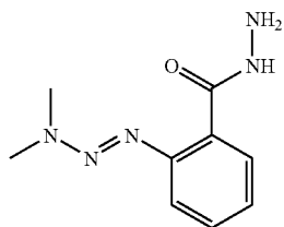
BENZOICACIDHYDRAZIDE033DIMETRIAZINO
