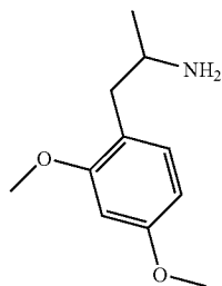
24DIMETHOXYAMPHETAMINE
