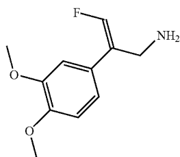
MDL72638
