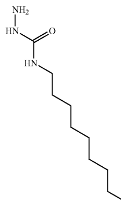
4DECYLSMICARBAZIDE
