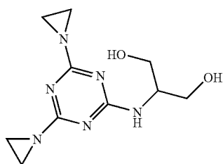
6BISHOCH2MEAMINO24DIAZIRIDINYLTRIAZINE
