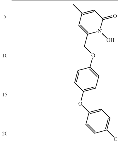
RILOPIROX
