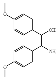
ISOLADOL
