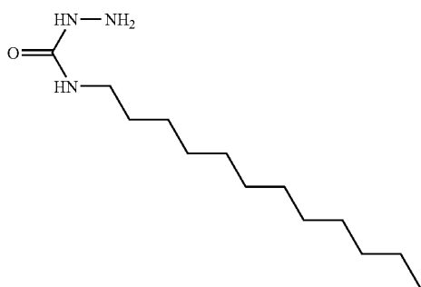
4DODECYLSEMICARBAZIDE
