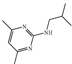
PYRIMIDINE21BUTYLAMINO46DIMETHYL
