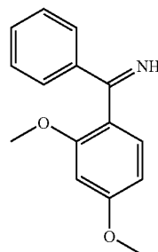
BENZENEMETHANIMINE24DIMETHOXYPHENYL
