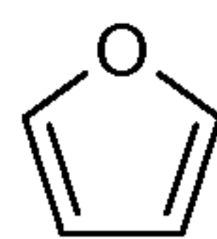
furan (furanyl)
