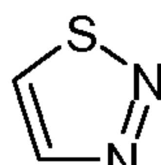
1-thia-2,3-diazole (1-thia-2,3-diazolyl)
