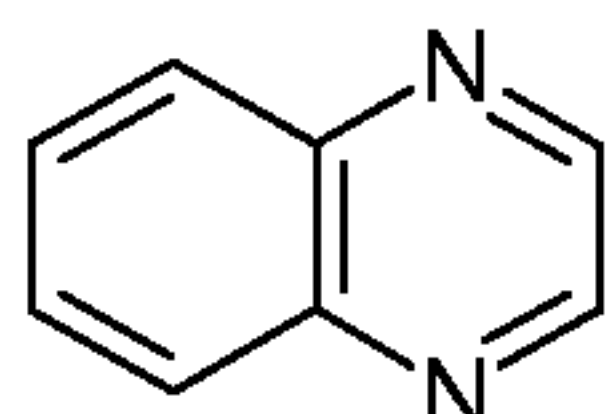
quinoxaline (quinoxalyl)
