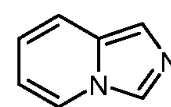
imidazo[1,5-a]pyridine (imidazo[1,5-a]pyridinyl)
