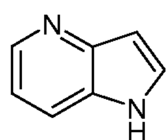
pyrrolo[3,2-b]pyridine (pyrrolo[3,2-b]pyridinyl)
