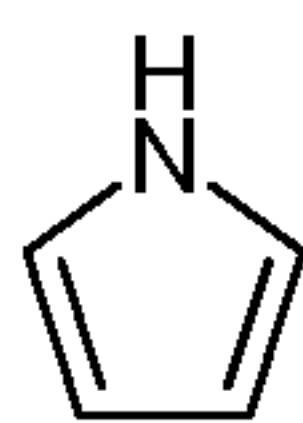
pyrrole (pyrrolyl)
