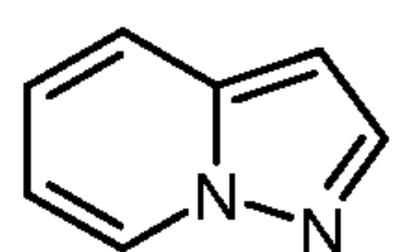
pyrazolo[1,5-a]pyridine (pyrazolo[1,5-a]pyridinyl)
