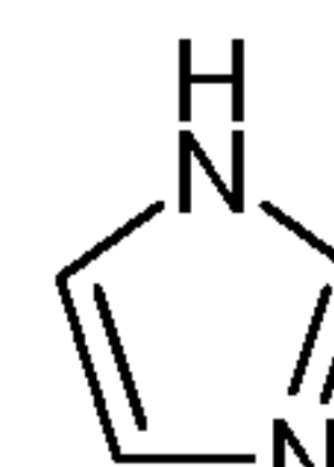
imidazole (imidazolyl)
