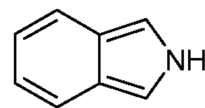
isoindole (isoindolyl)
