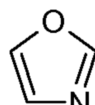
oxazole (oxazolyl)
