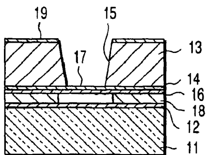
FIG. 8A PRIOR ART
