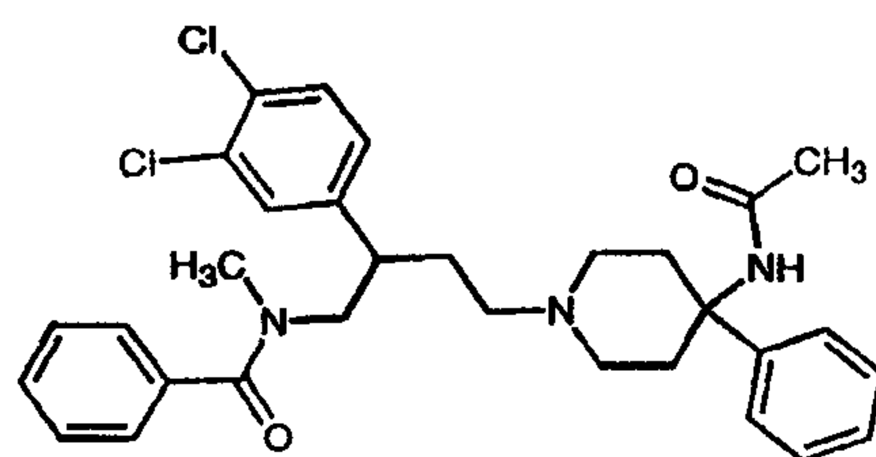
SR-48968 (37)
