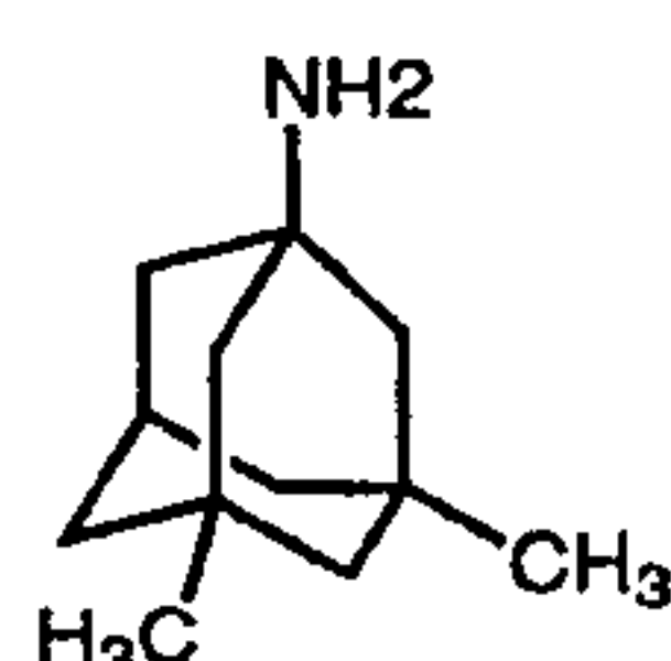
Memantine (5)
