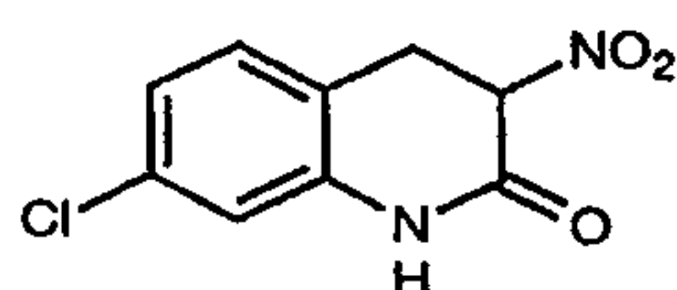
L-698,544 (23)
