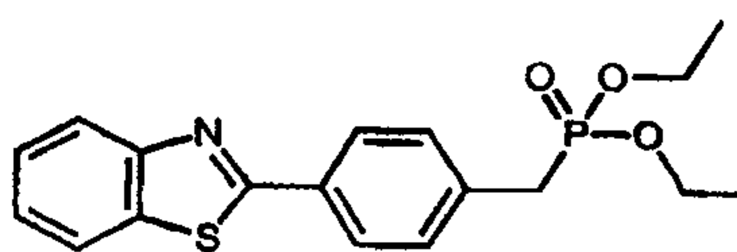
Fostedil (75)
