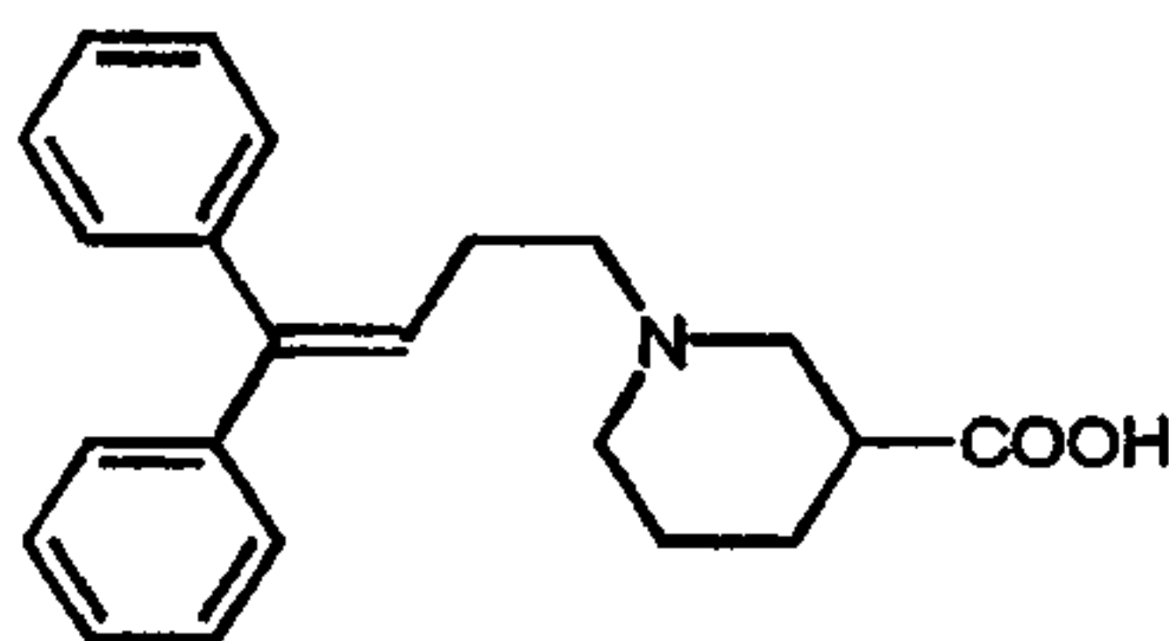
SKF 89976-A (53)
