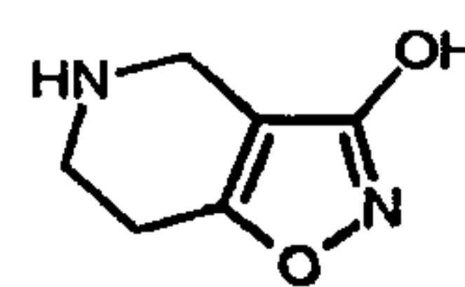
THPO (52)
