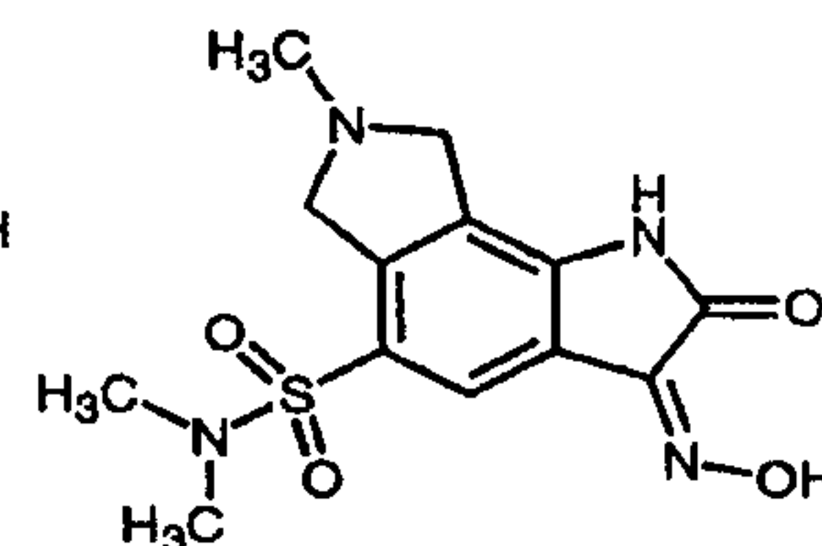
NS-257 (26)
