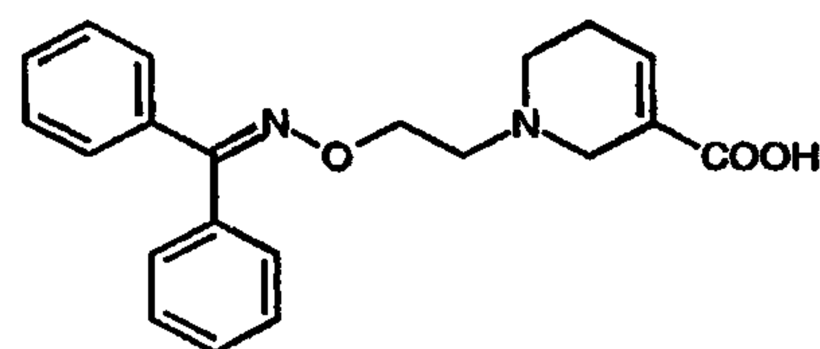
NO-711 (54a)
