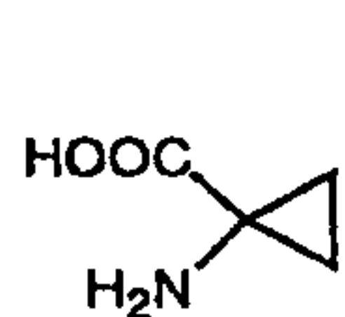
ACPC (15)
