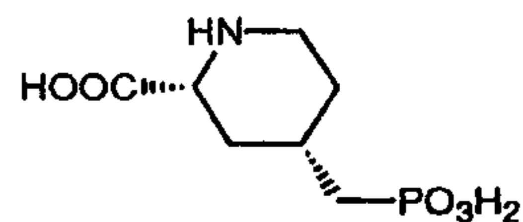
CGS 19755 (1)
