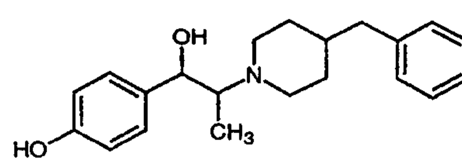
Ifenprodil (10)
