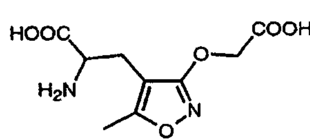
AMOA (25)
