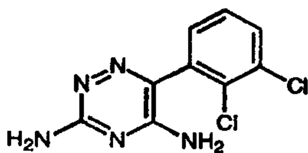
Lamotrigine (65)
