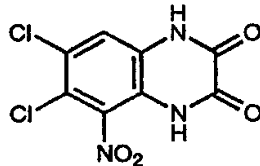
ACEA1021 (17)
