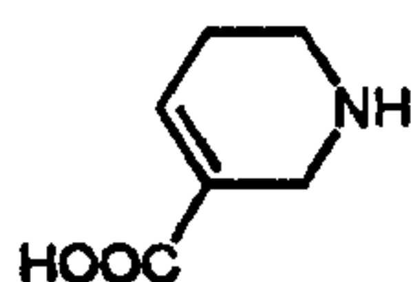
Guvacine (51)
