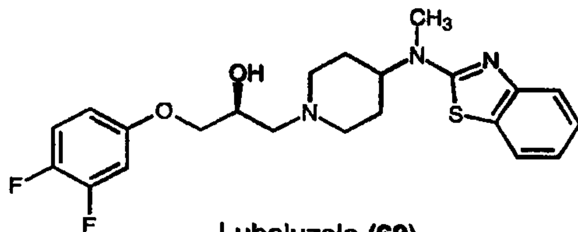
Lubeluzole (68)
