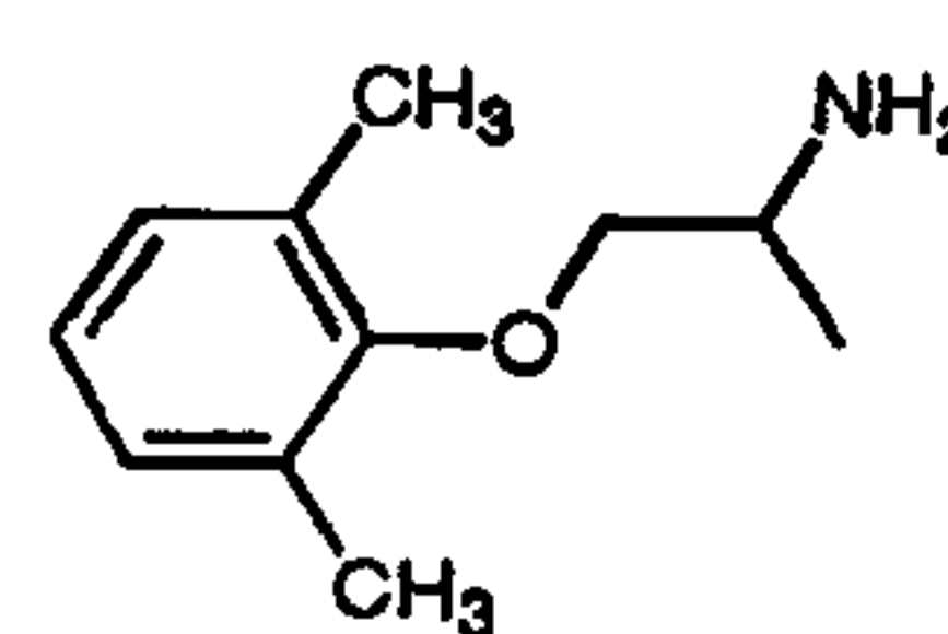
Mexiletene (73)
