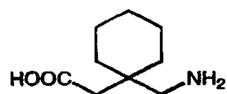
Gabapentin (46)
