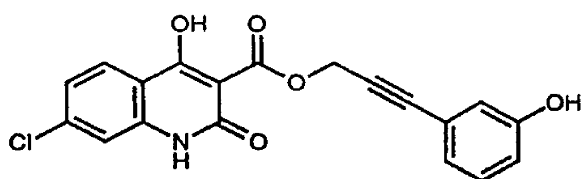
L-701,273 (14b)
