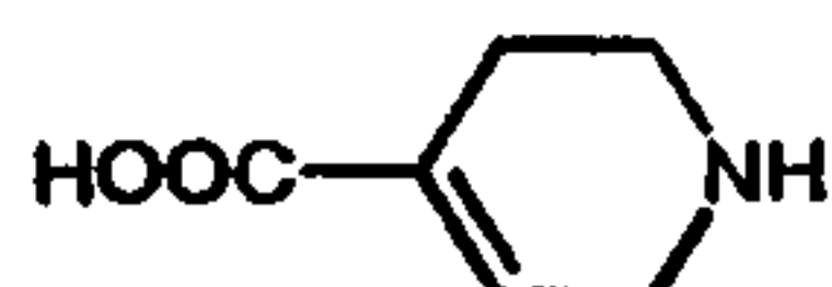
Isoguvacine (48)
