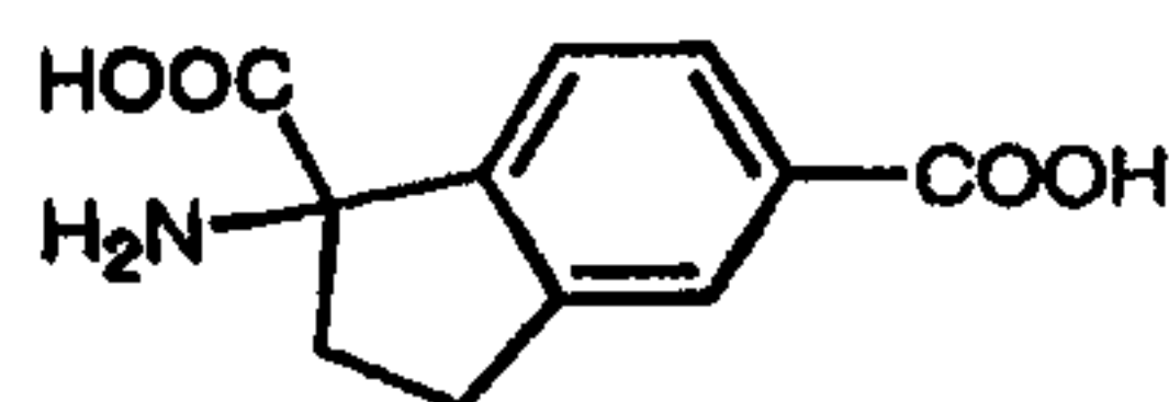
UPF523 (31)
