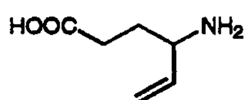
Vigabatrin (55)
