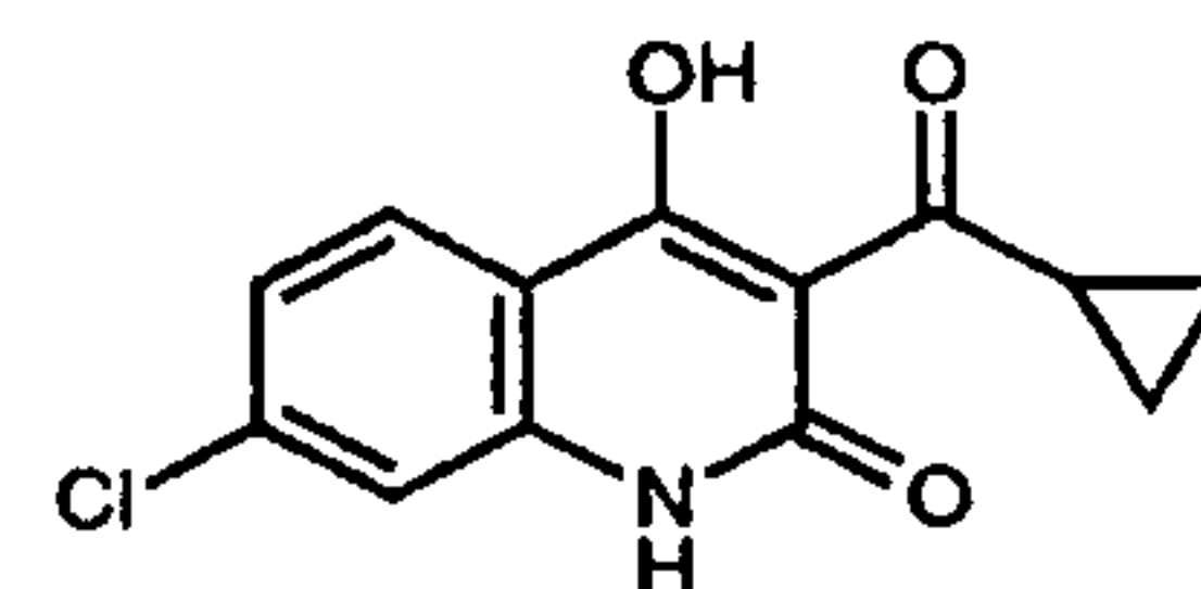
L-701,252 (14a)
