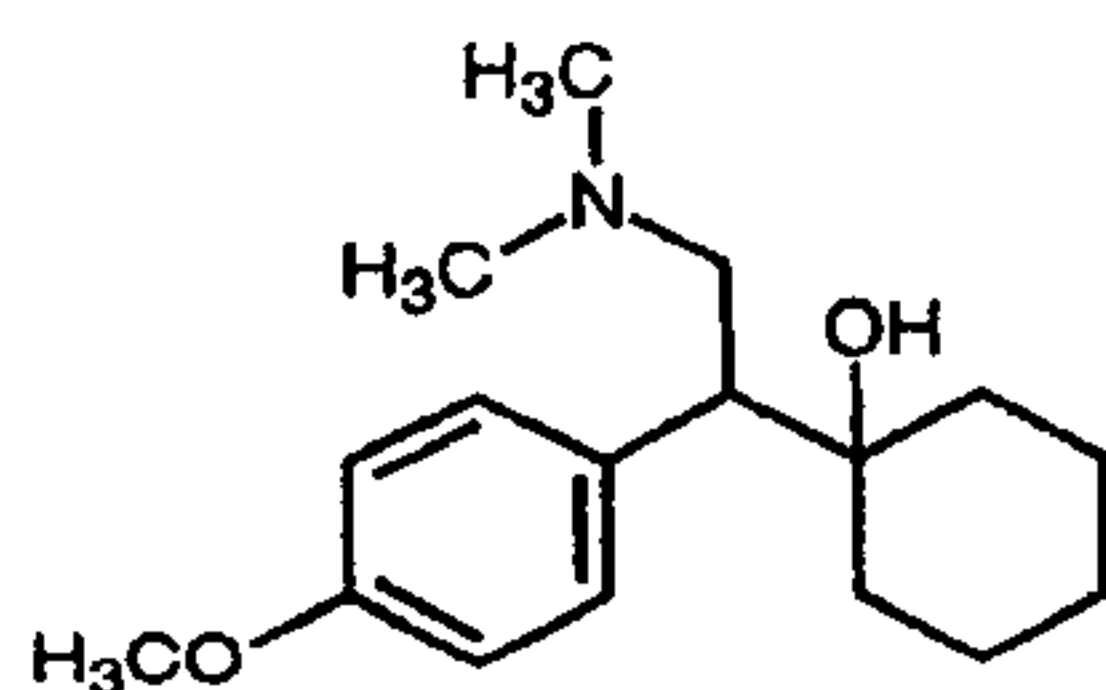
Venlafaxine (4f)
