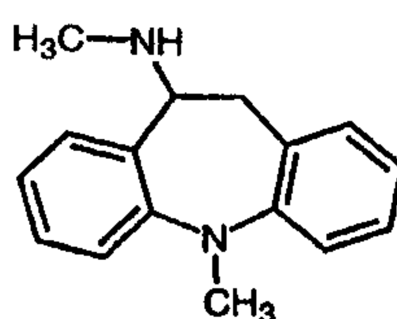
Metapramine (4a)
