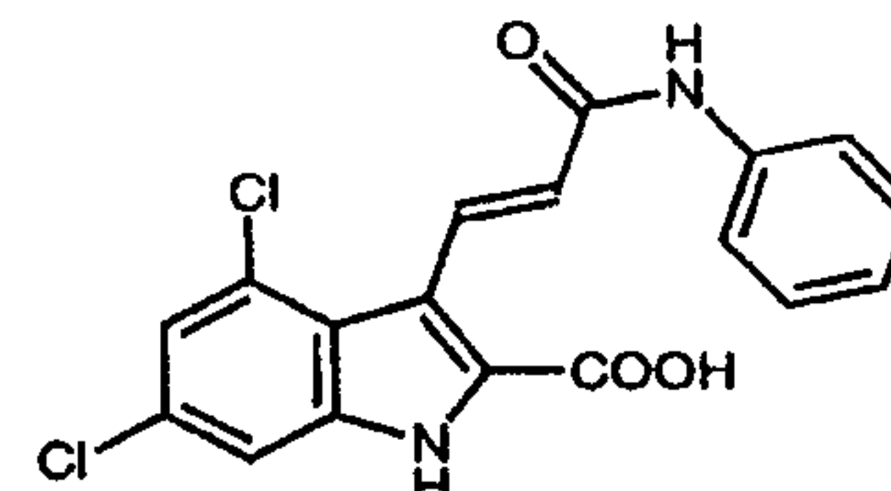
GV150526A (14d)
