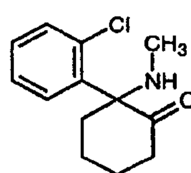
Ketamine (6)
