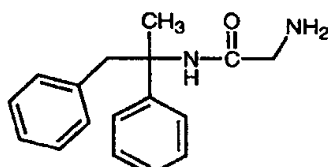
Remacemide (9)
