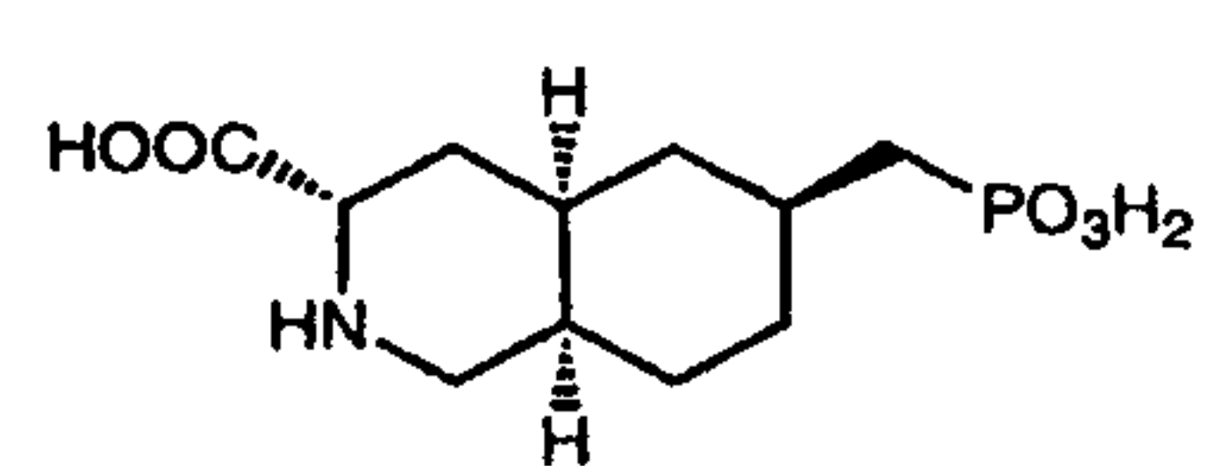
LY 235959 (3a)
