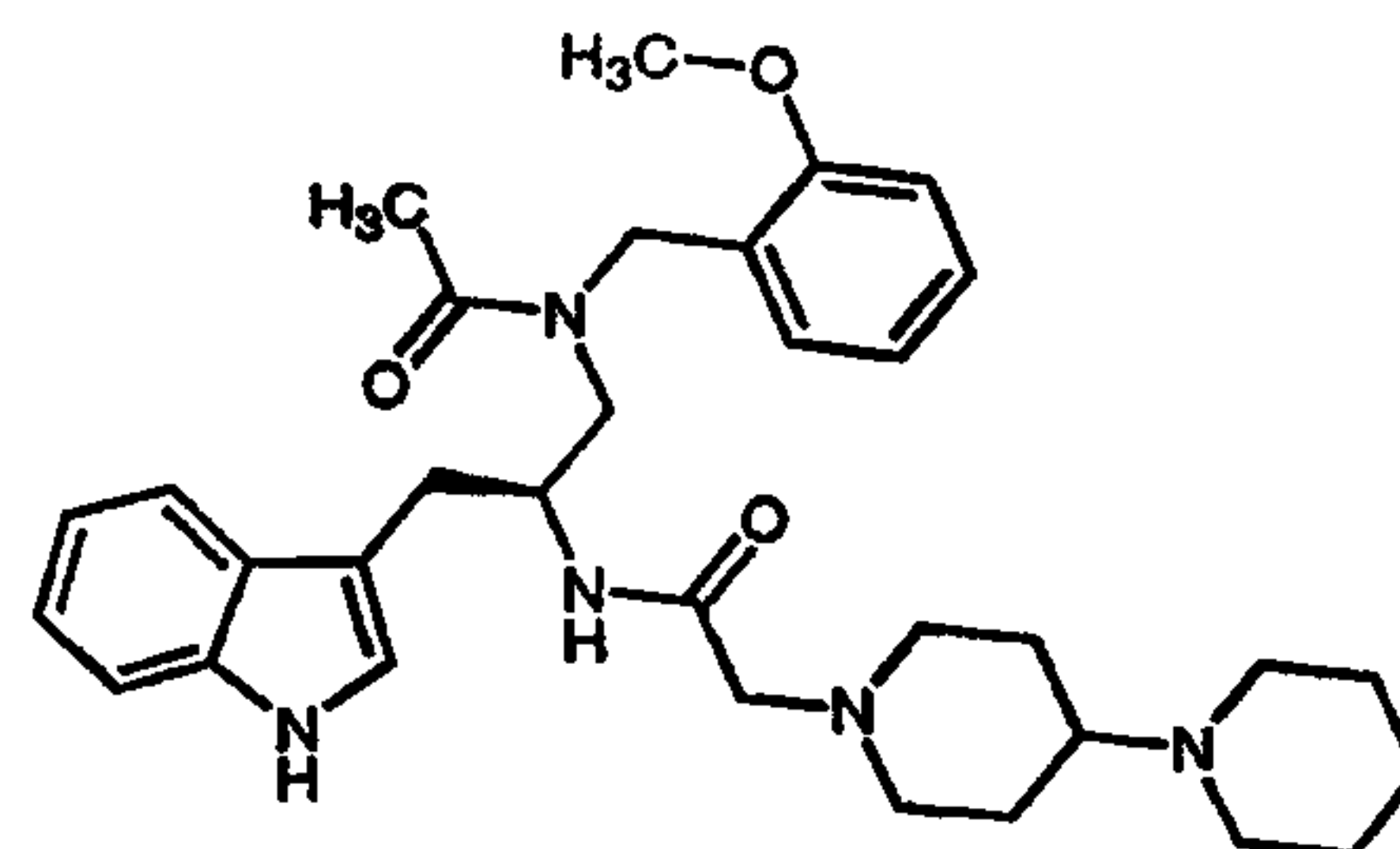
LY 303870 (34)
