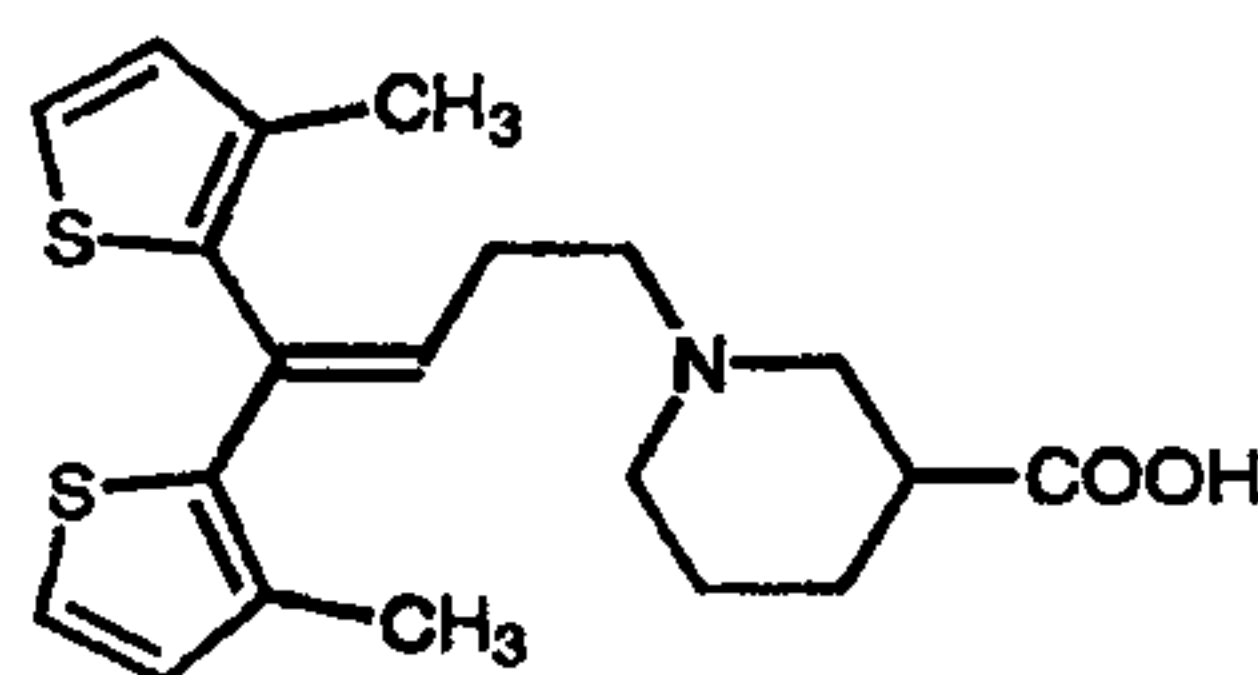
Tiagabine (54)
