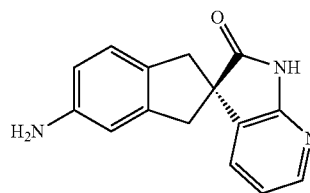
(R)-5-Amino-1,3-dihydrospiro[indene-2,3'-pyrrolo[2,3-b]pyridin]-2'(1'H)-one
