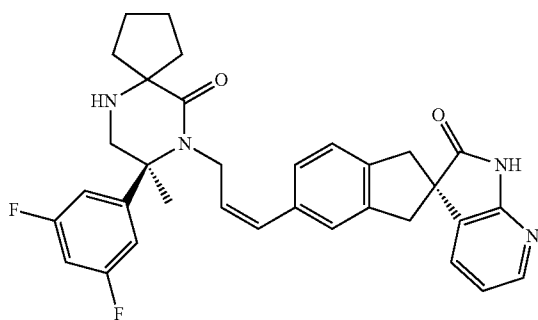
(2R)-5-{(1Z)-3-[(8S)-8-(3,5-Difluorophenyl)-8-methyl-10-oxo-6,9-diazaspiro[4.5]dec-9-yl]prop-1-en-1-yl}-1,3-dihydrospiro[indene-2,3'-pyrrolo[2,3-b]pyridin]-2'(1'H)-one
