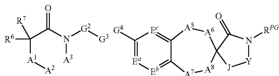
Ia
