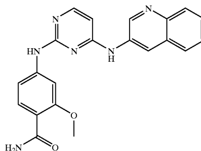
2-(Methoxy)-4-((4-(3-quinolinylamino)-2-pyrimidinyl)amino)benzamide
