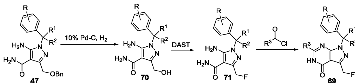
Scheme 27.
