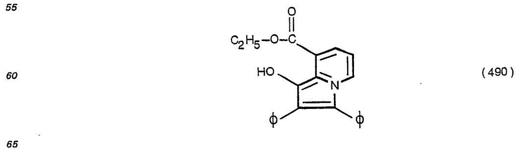
55 8-carboethoxy-2,3-diphenyl-1-indolizinol
