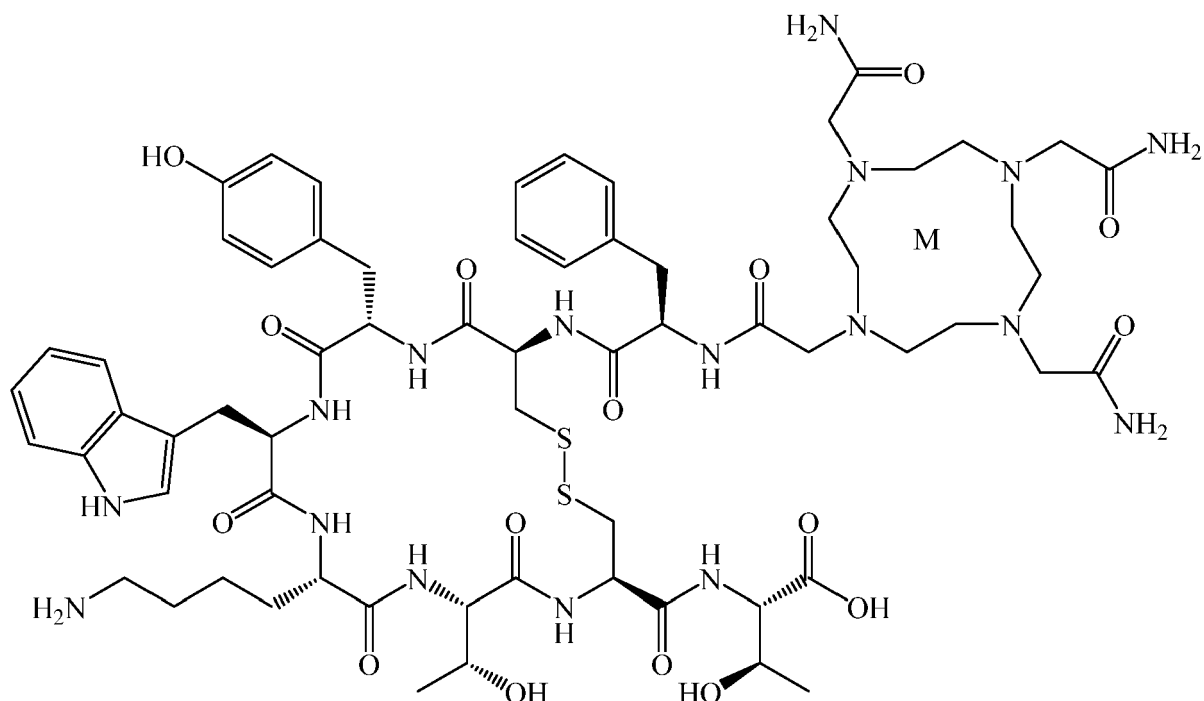
“DOTAMTATE”,
