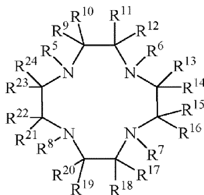
Formel (V)
