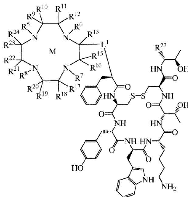
Formel (VIII),
