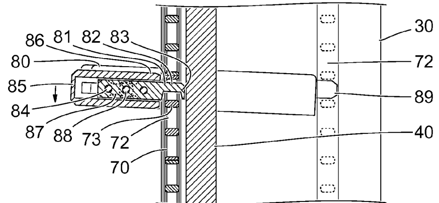
Fig. 6 A-A
