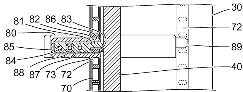
Fig. 9 A-A
