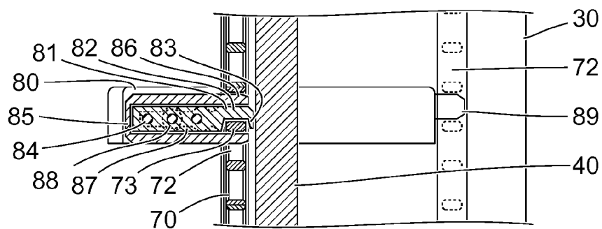
Fig. 9 A-A
