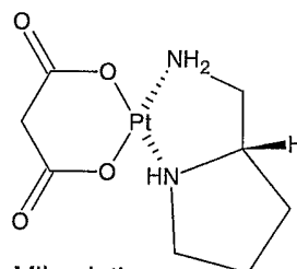
Miboplatin
