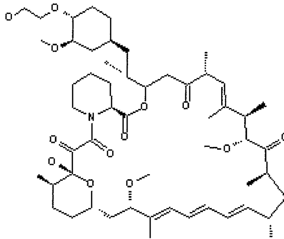
Everolimus
