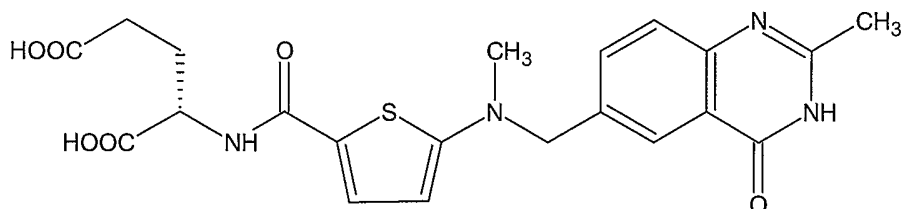
Tomudex.
