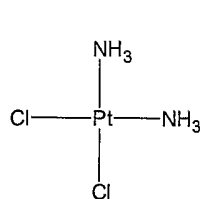
Cisplatin
