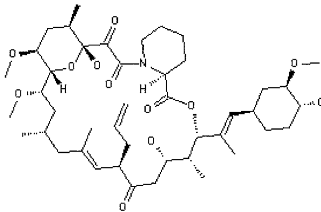
Tacrolimus
