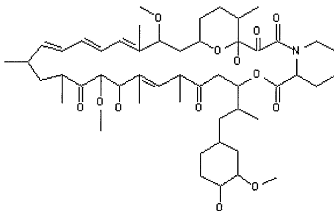
Sirolimus
