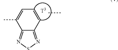
(V)
