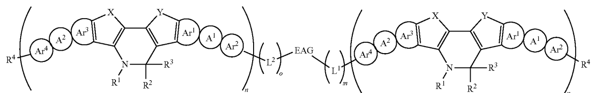
formula (Ij)
