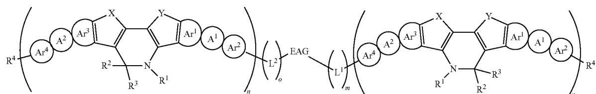
formula (Ik)
