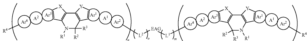
formula (Ik)
