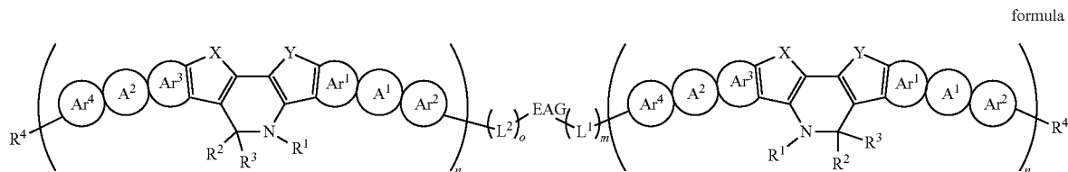
formula (Ik)
