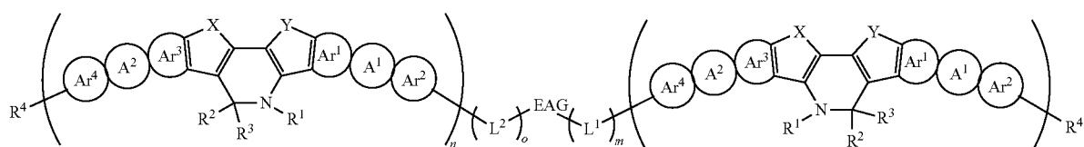
formula (Ik)
