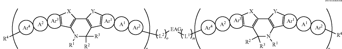
formula (Ij)
