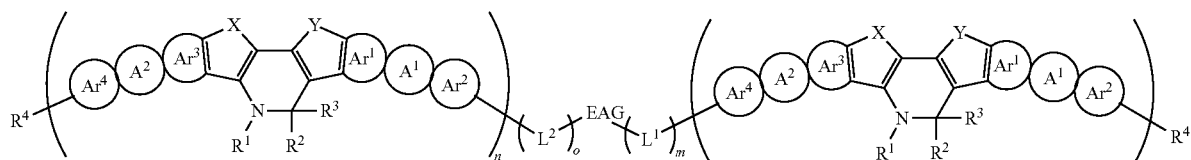
formula (Ij)
