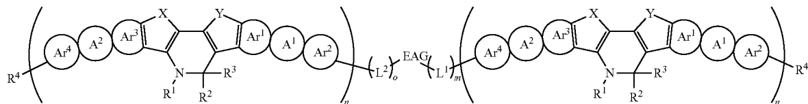
formula (Ij)
