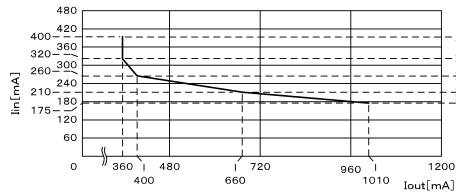
(b) TA点の入力電流Iin及びTB点の出力電流Iout
