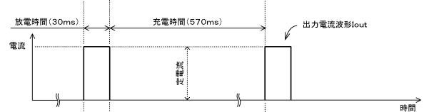
(c) 最大出力時におけるTB点の出力電圧の波形
