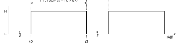
(e) TD点の論理
