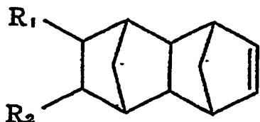
Allgemeine Formel (3)
