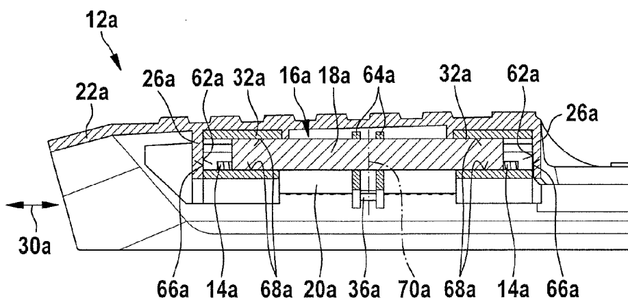
Fig. 4 (Section A-A)
