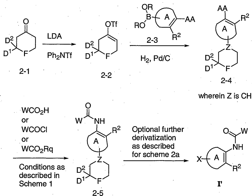
Scheme 2a
