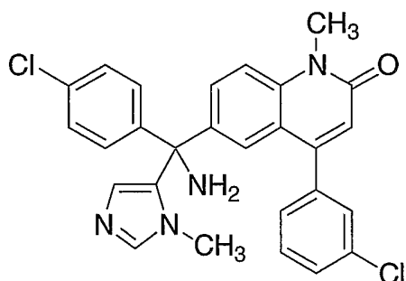
FTI - Tipifarnib
