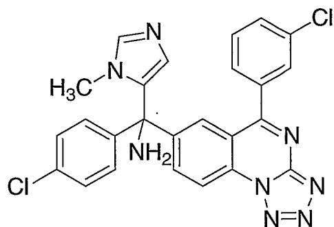
FTI - 176
