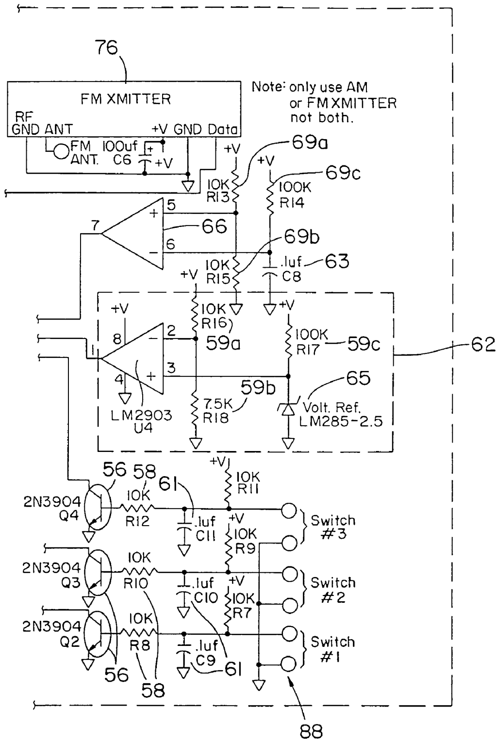
FIG. 3A-2
