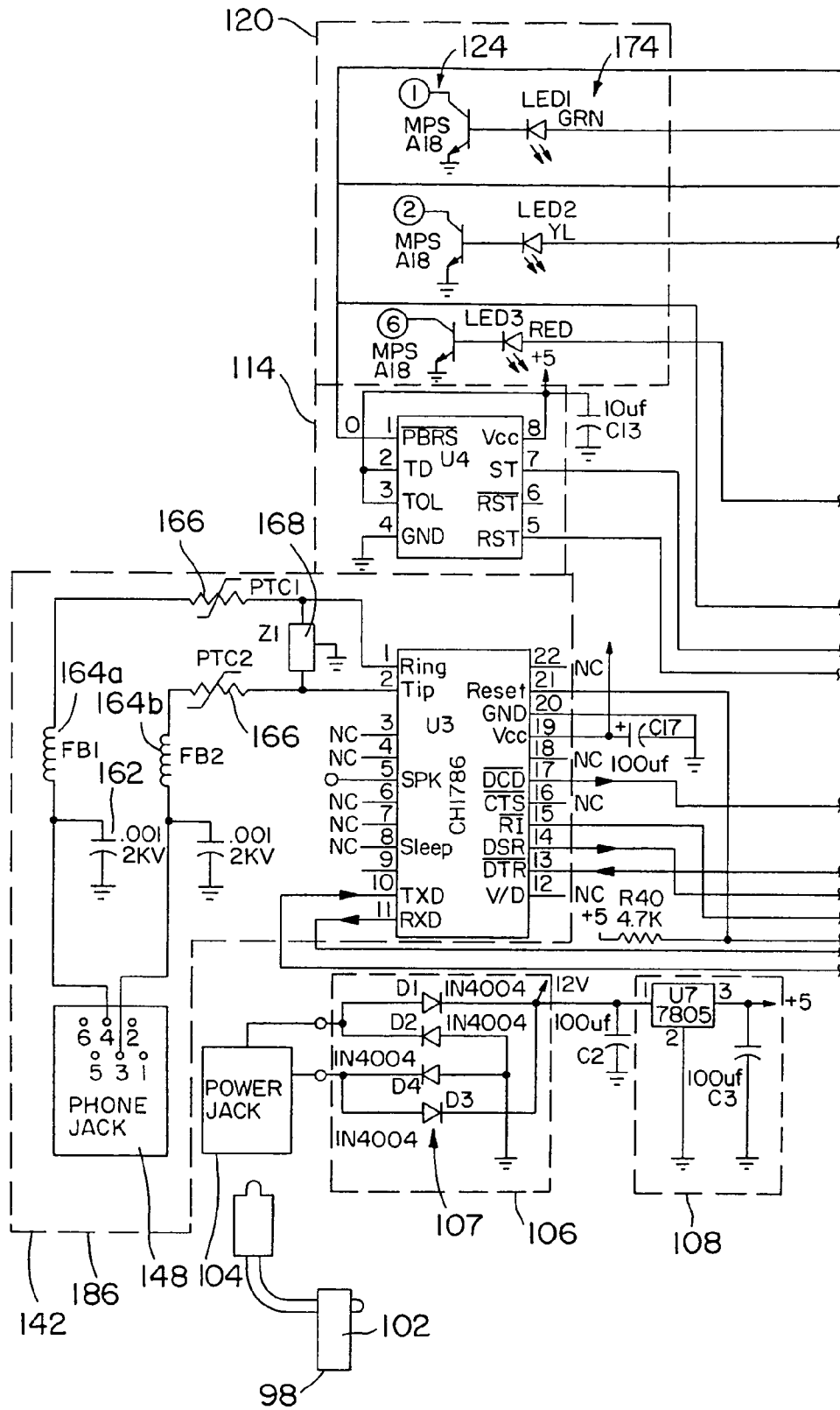
FIG. 3B-1
