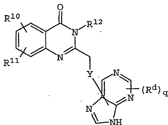
(IV)
