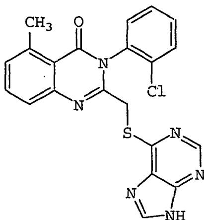
D-026
