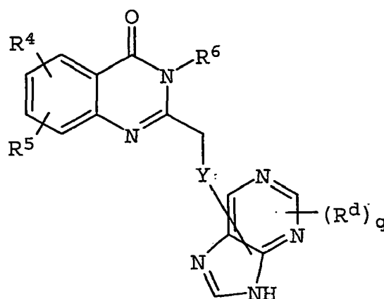
(II)
