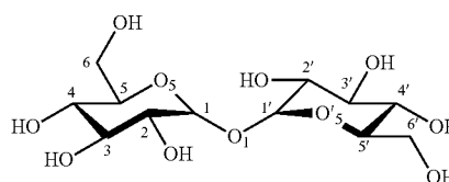
\alpha,\alpha -Trehalose
