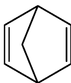
norbornadiene
