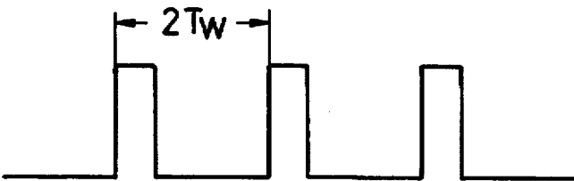
FIG. 16C
