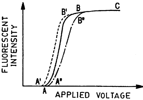
FIG. 17C
