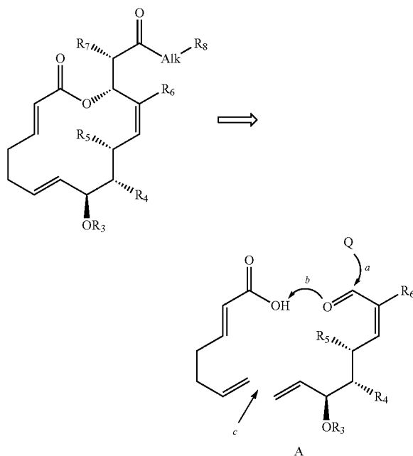
Scheme 1A
